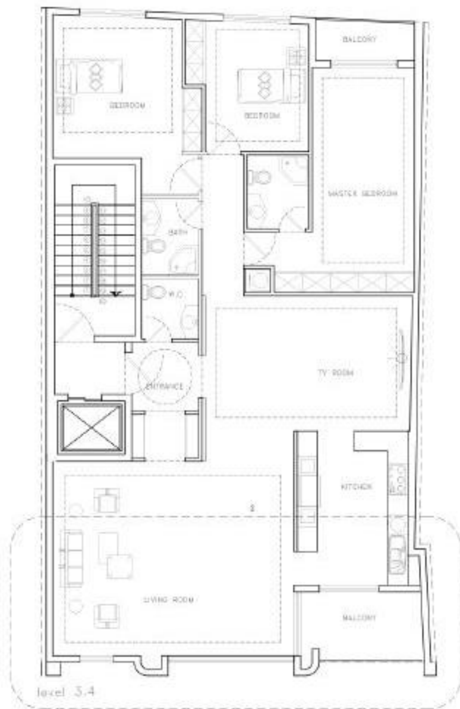
پلان جداره نمای جنوبی ( طبقه سوم و چهارم )
