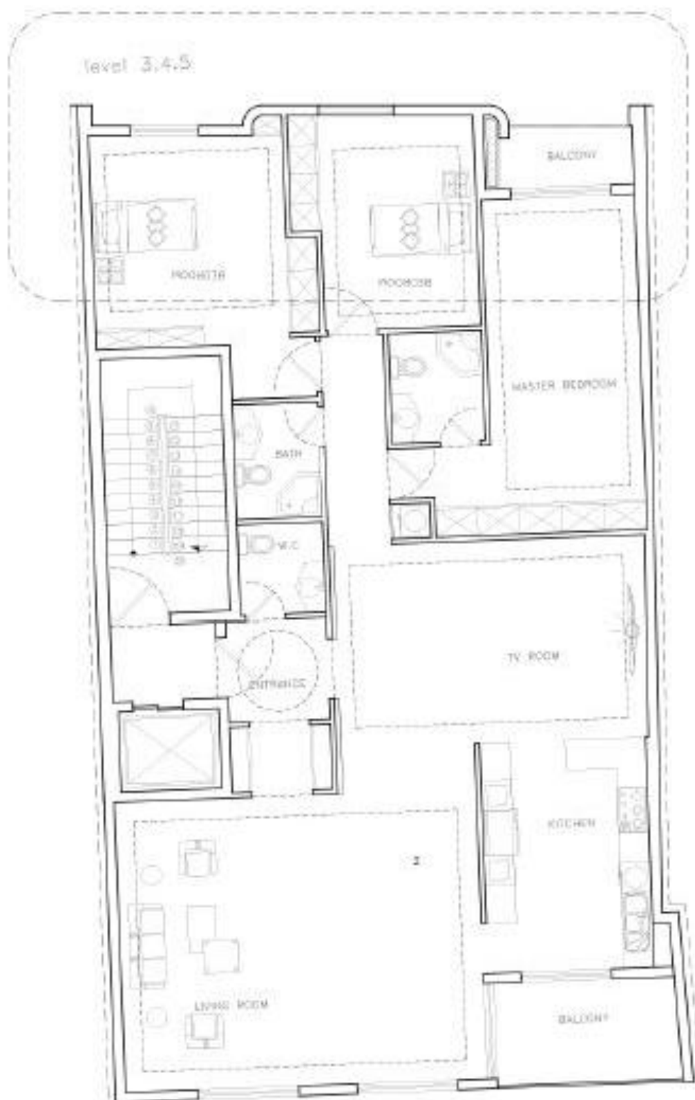
پلان جداره نمای اصلی ( طبقه سوم ، چهارم ، پنجم )
