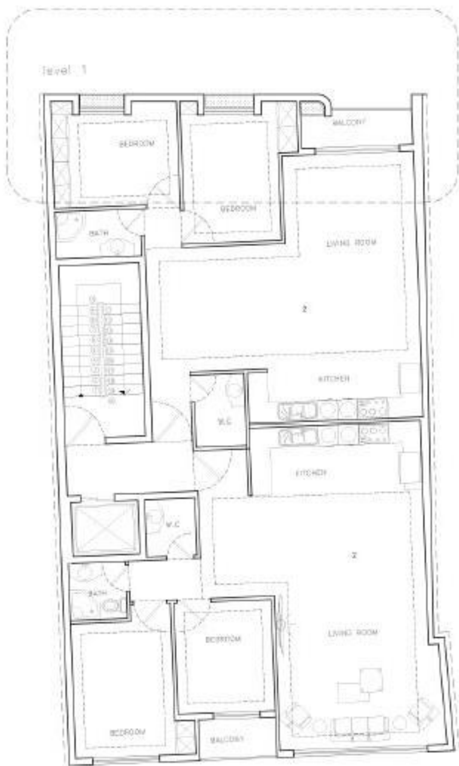
پلان جداره نمای اصلی (طبقه اول)
