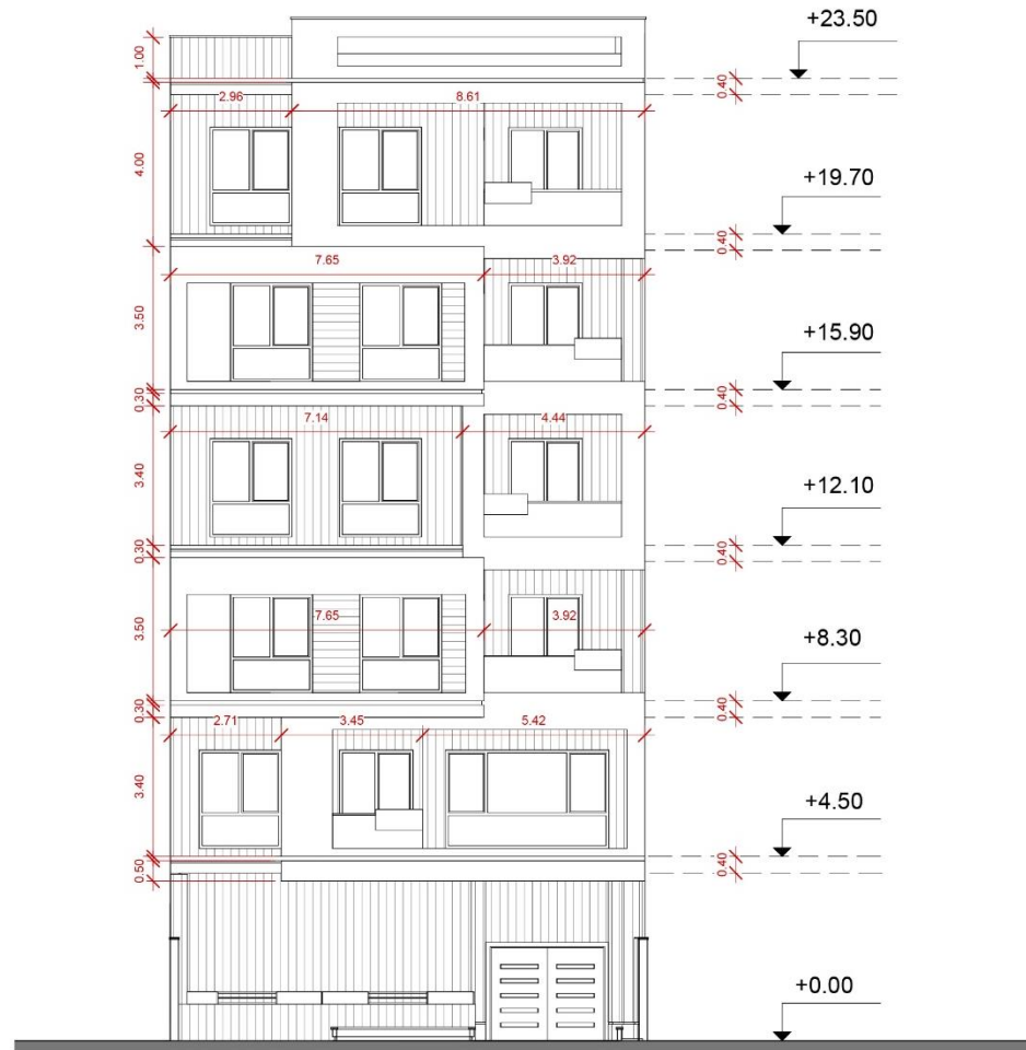
نمای جنوبی | اندازه گذاری
