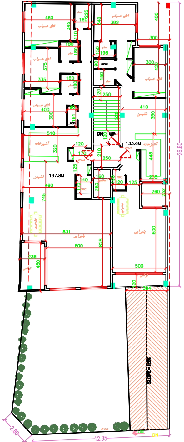
پلان طبقه ۳-۴-۵
