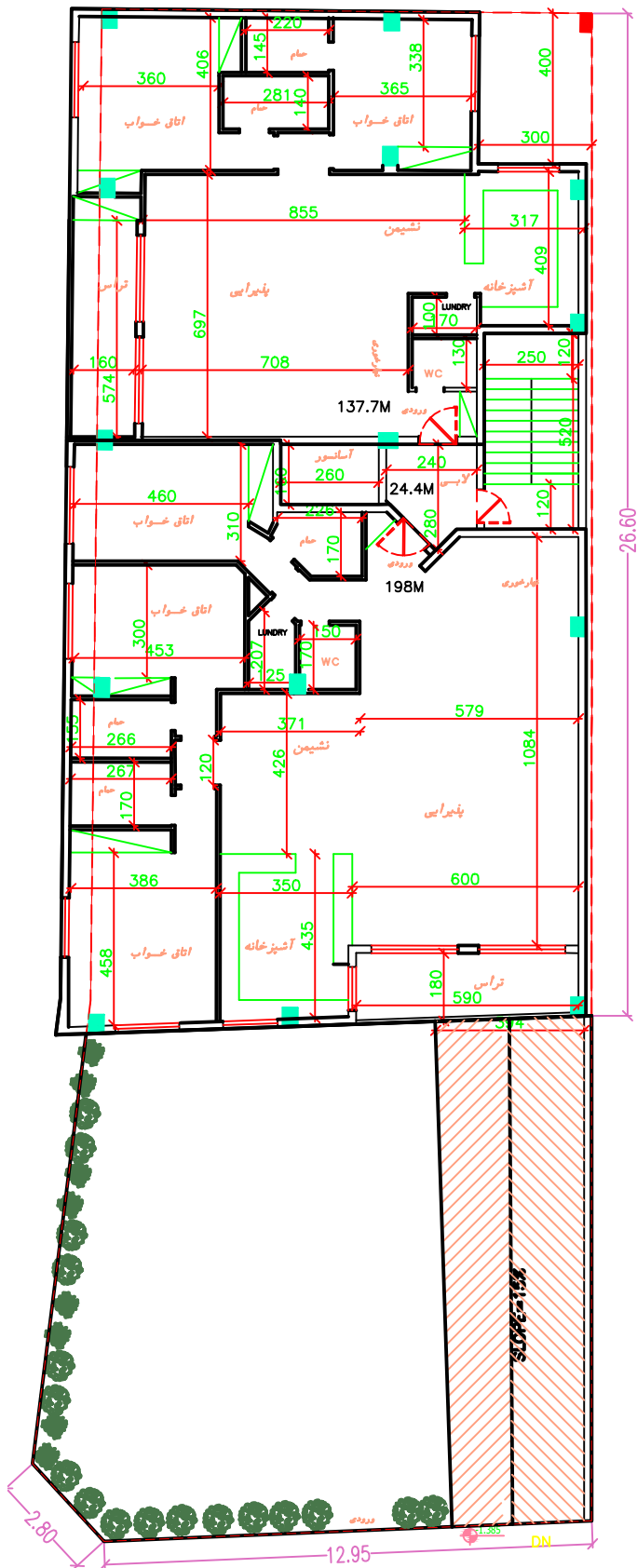
پلان طبقه ۵-۱
