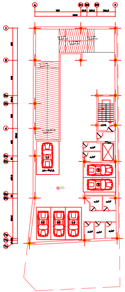
پلان زیر زمین دوم
