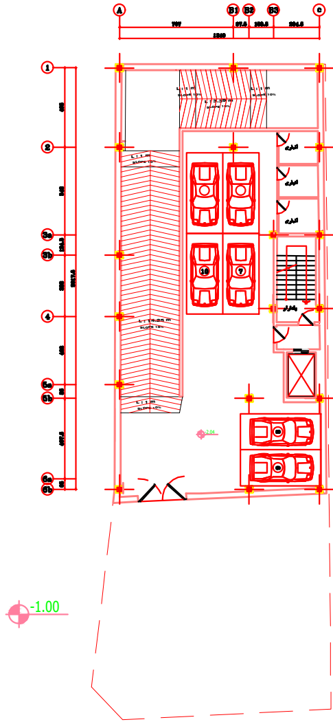
پلان زیرزمین اول
