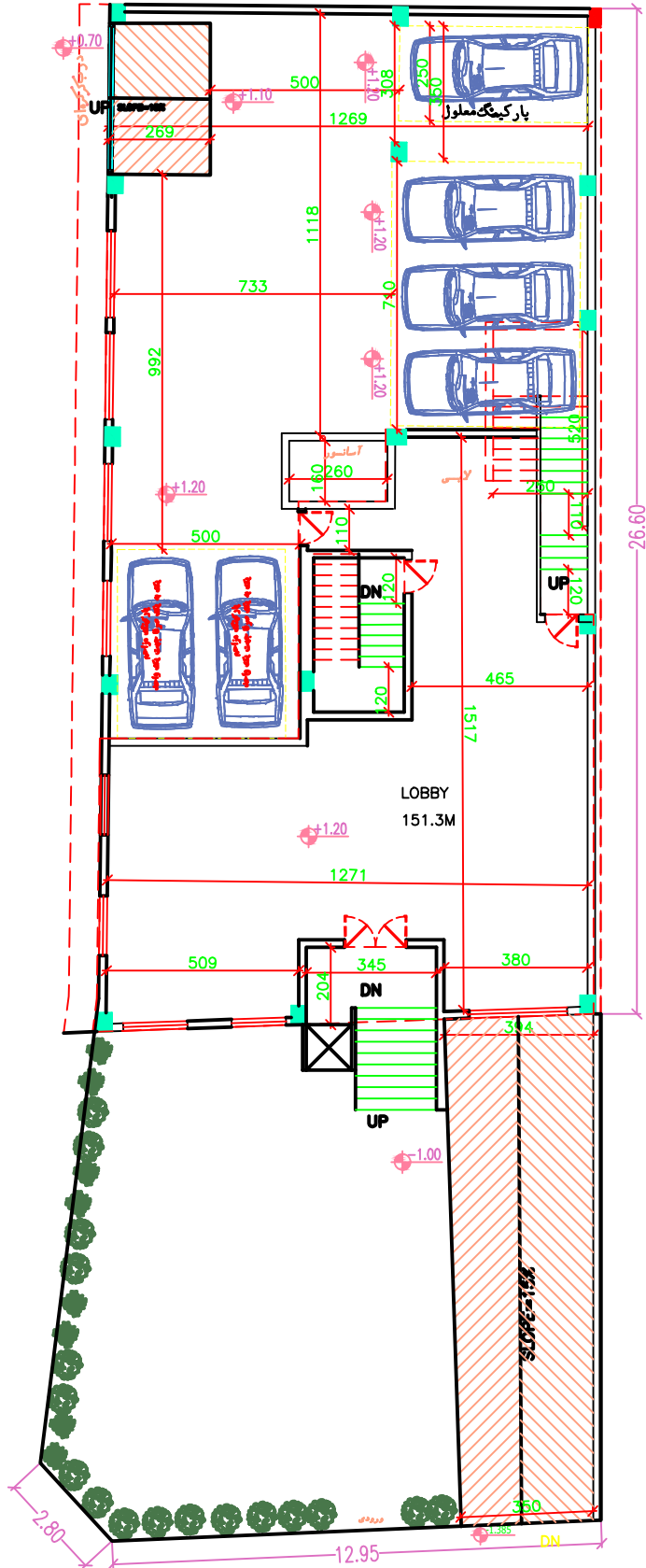
پلان همکف شماره ۱۰۰
