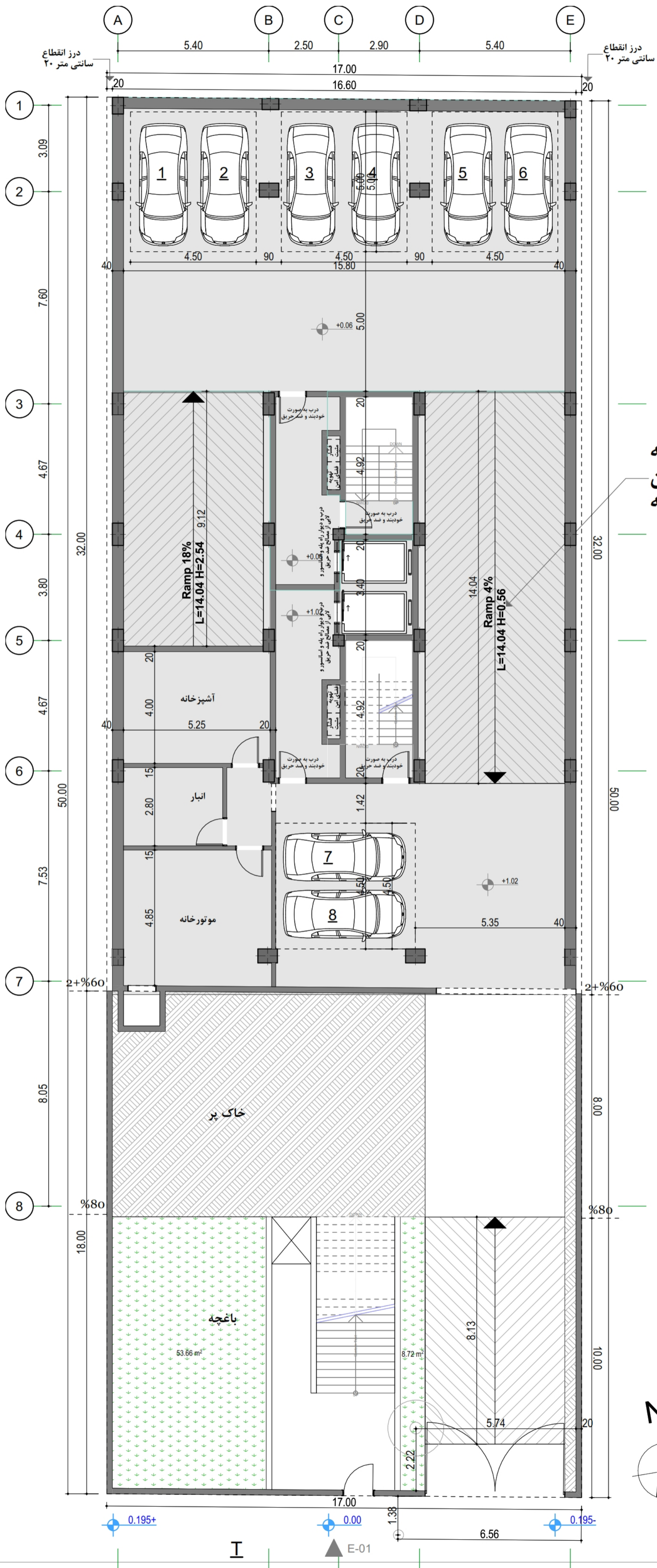
پلان زیرزمین اول
