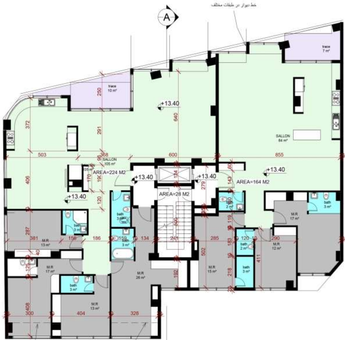
پلان اندازه گذاری پلان تیب طبقات
