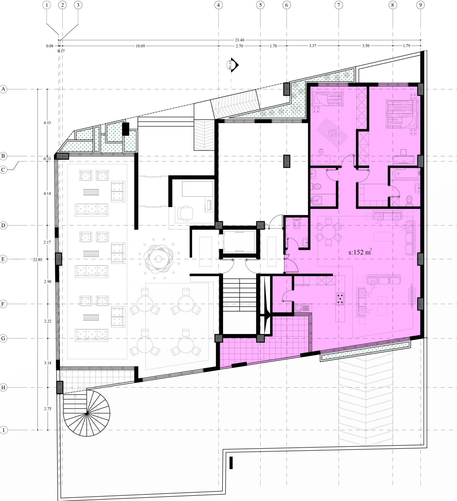
پلان مبلمان همکف
