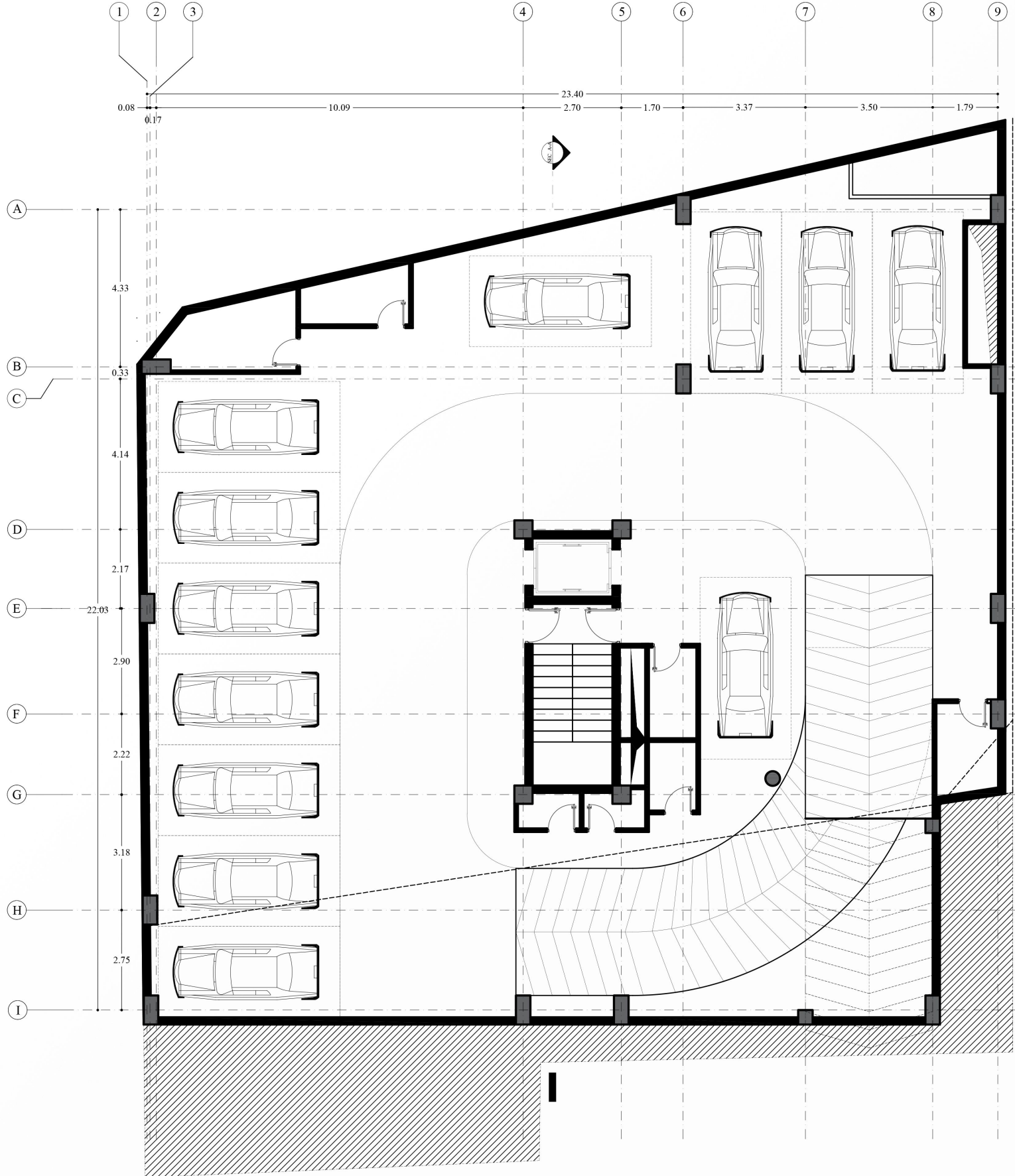
پلان مبلمان زیر زمین ۲-
