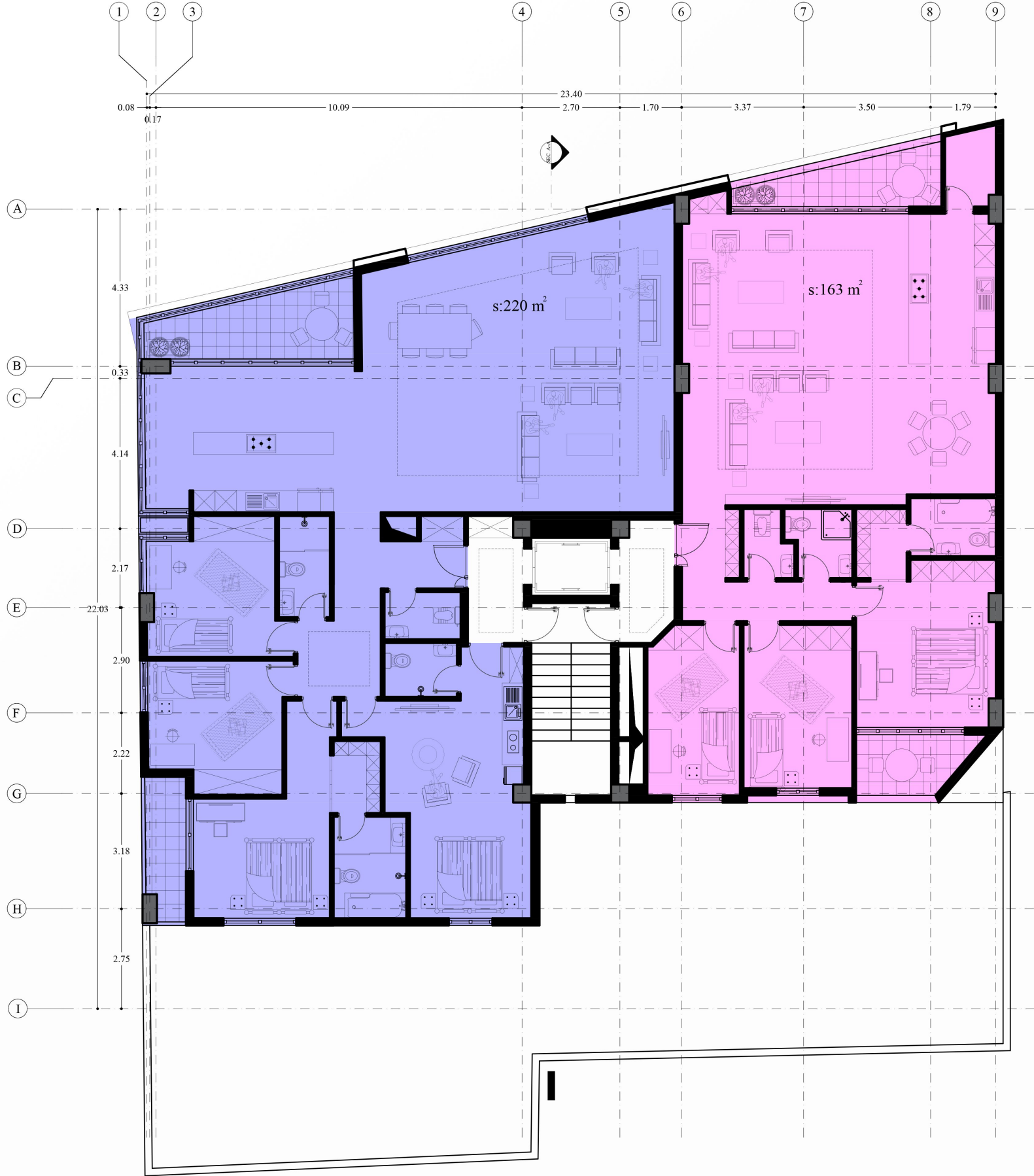
پلان مبلمان طبقه ششم
