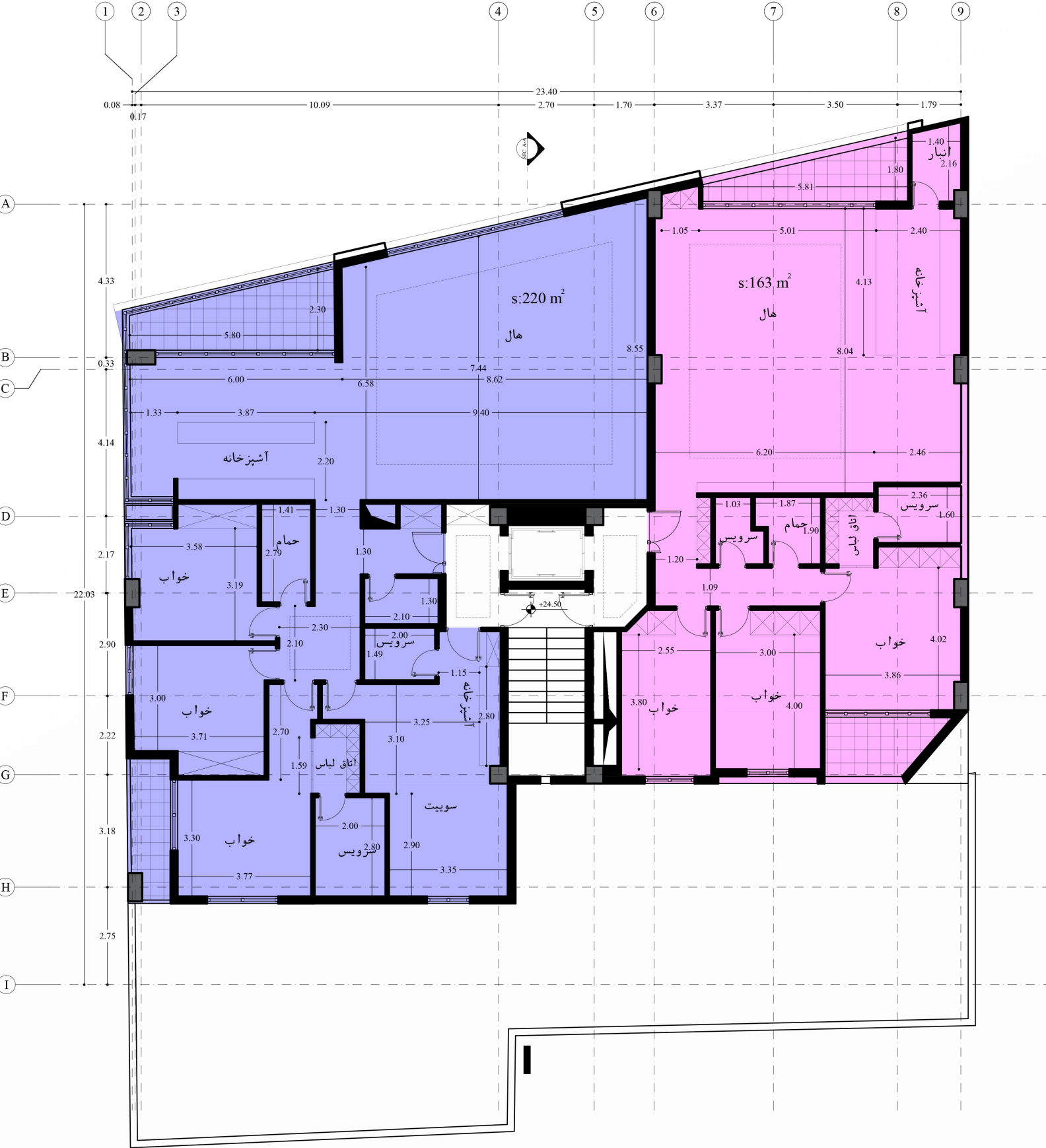
پلان اندازه گذاری طبقه ششم
