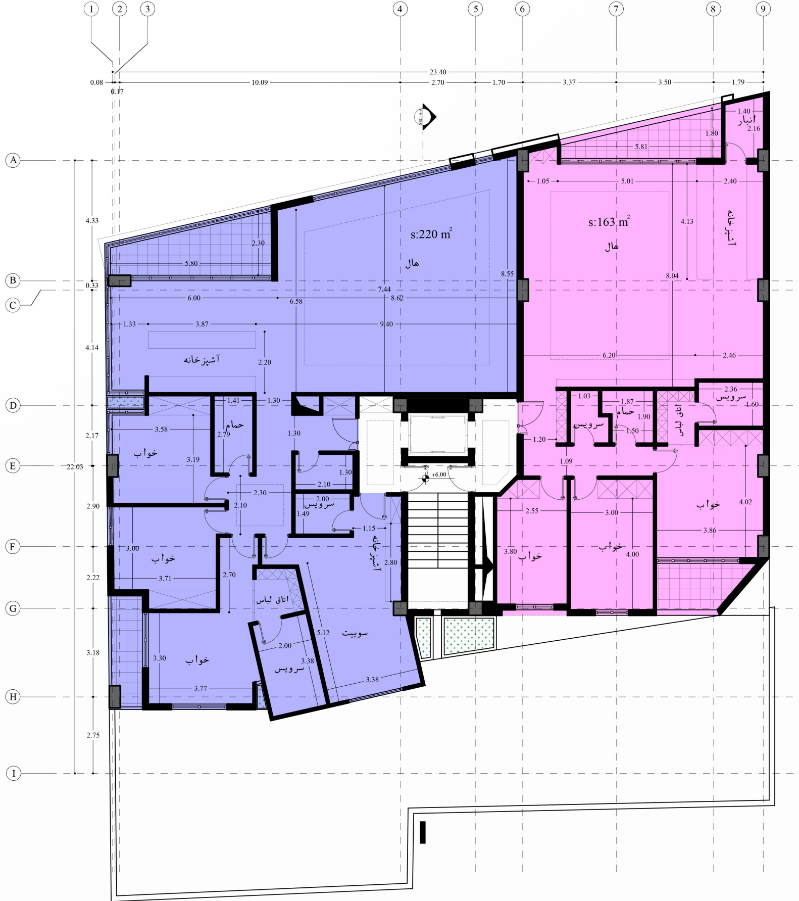
پلان اندازه گذاری طبقه اول
