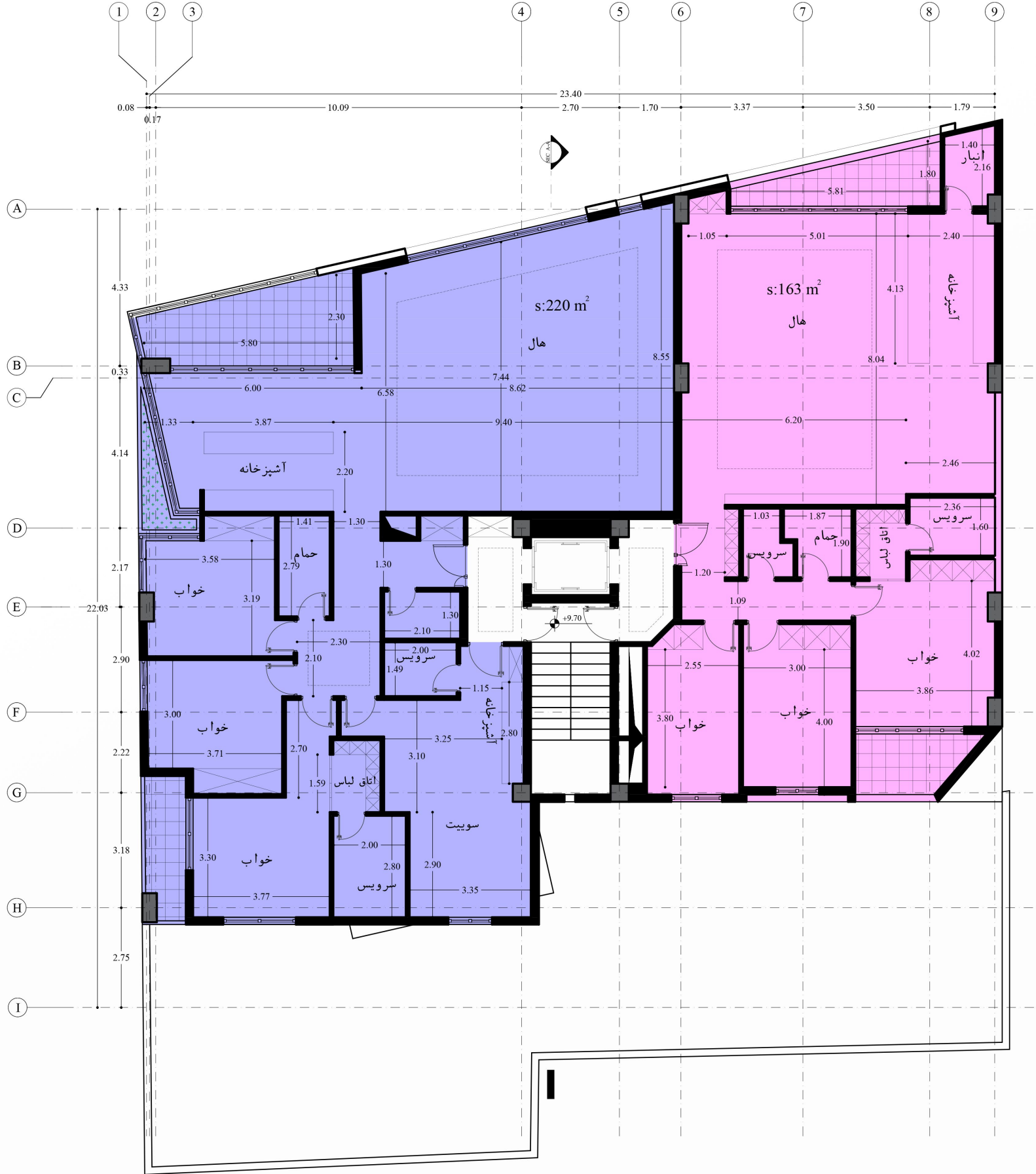
پلان اندازه گذاری طبقه دوم
