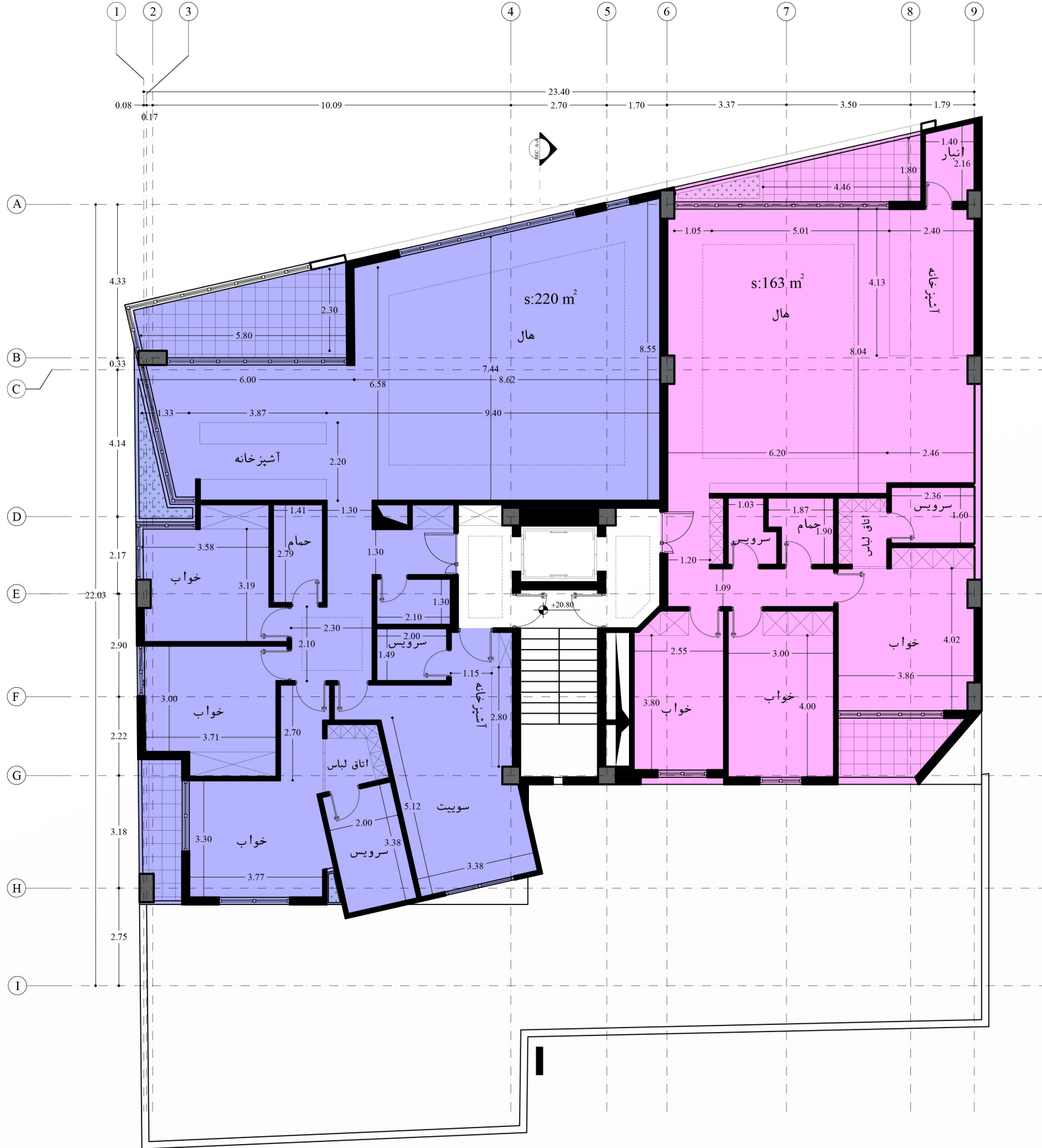
پلان اندازه گذاری طبقه پنجم
