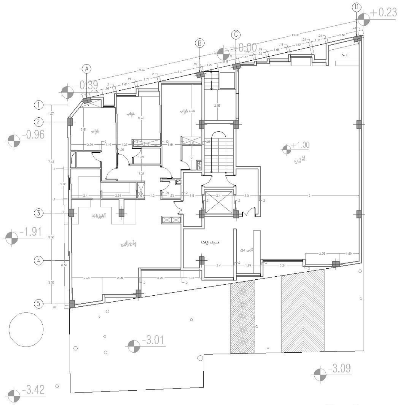
پلان همکف مقیاس: 1:100
