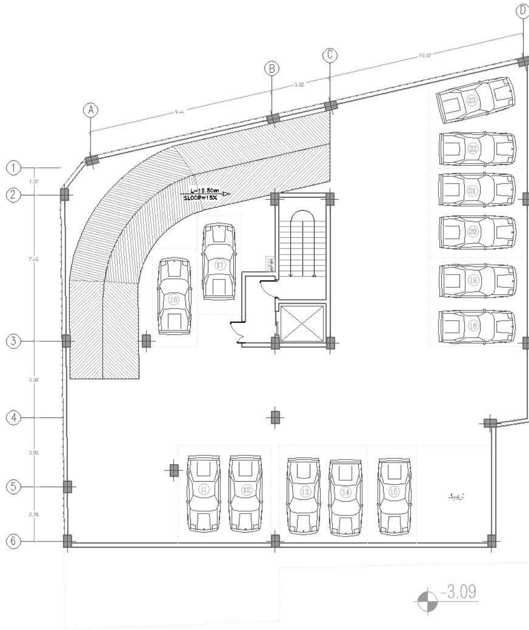
پلان زیرزمین ۳- مقیاس: ۱:۱۰۰
