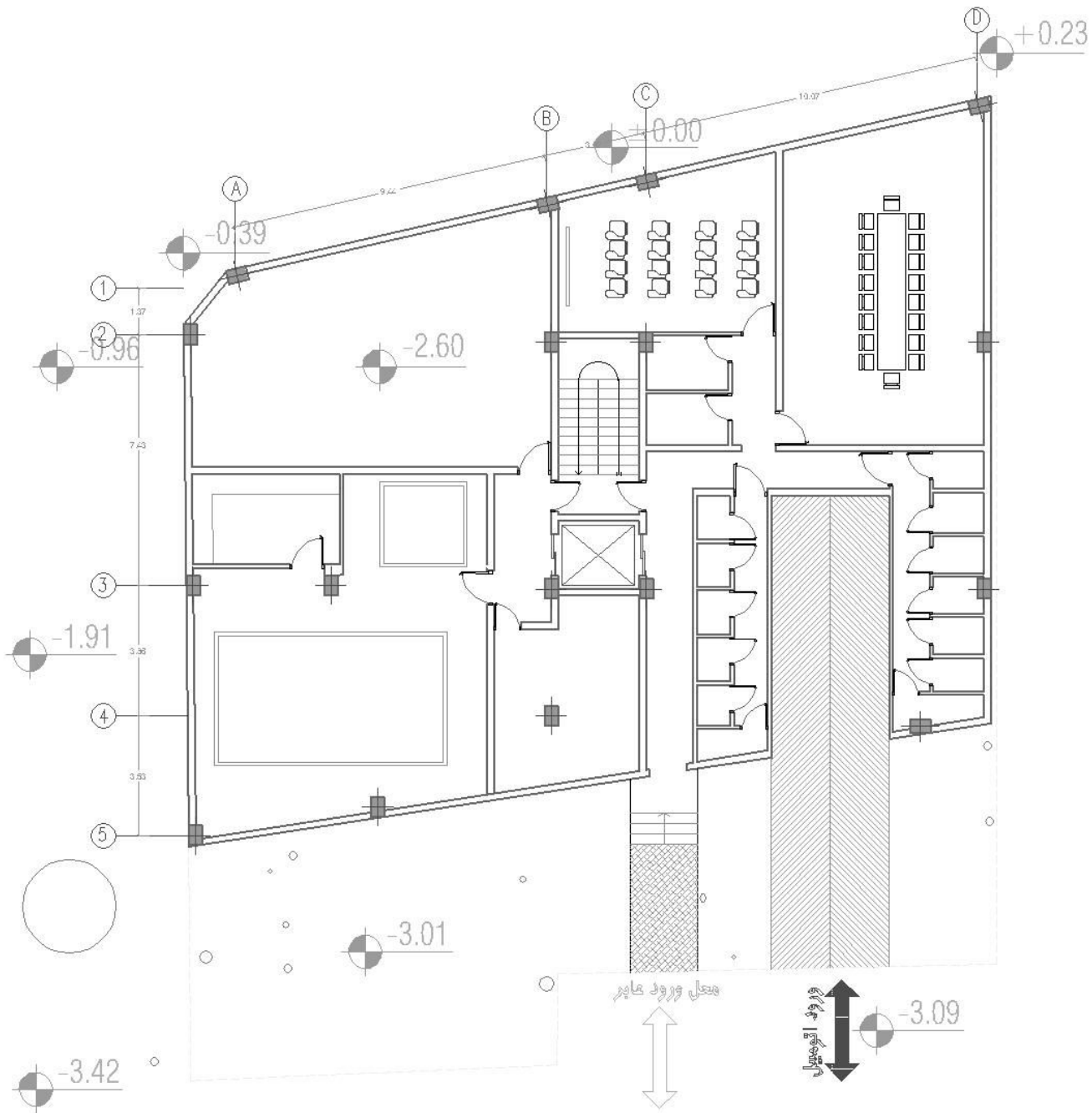
پلان زیرزمین ۱- مقیاس: ۱:۱۰۰
