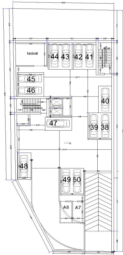
basement -4
