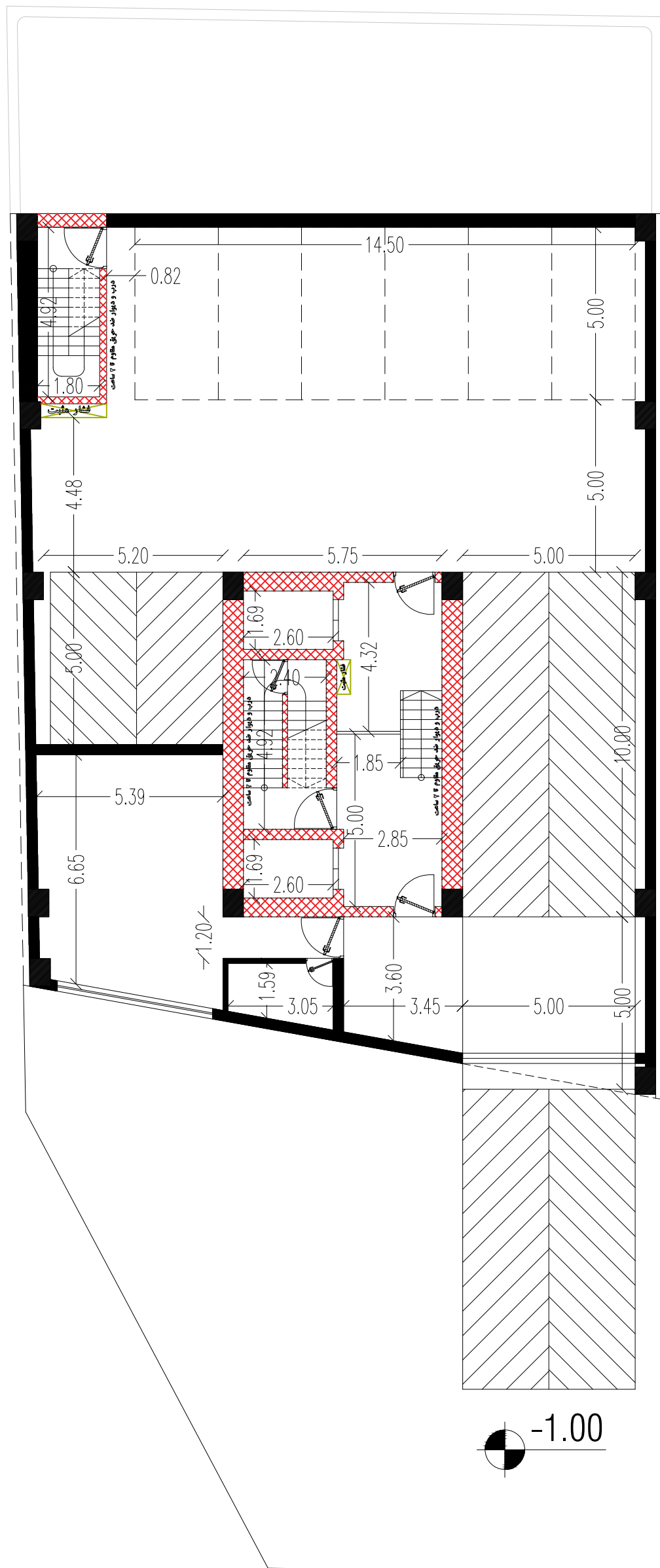
پلان اندازه گذاری زیر زمین اول
