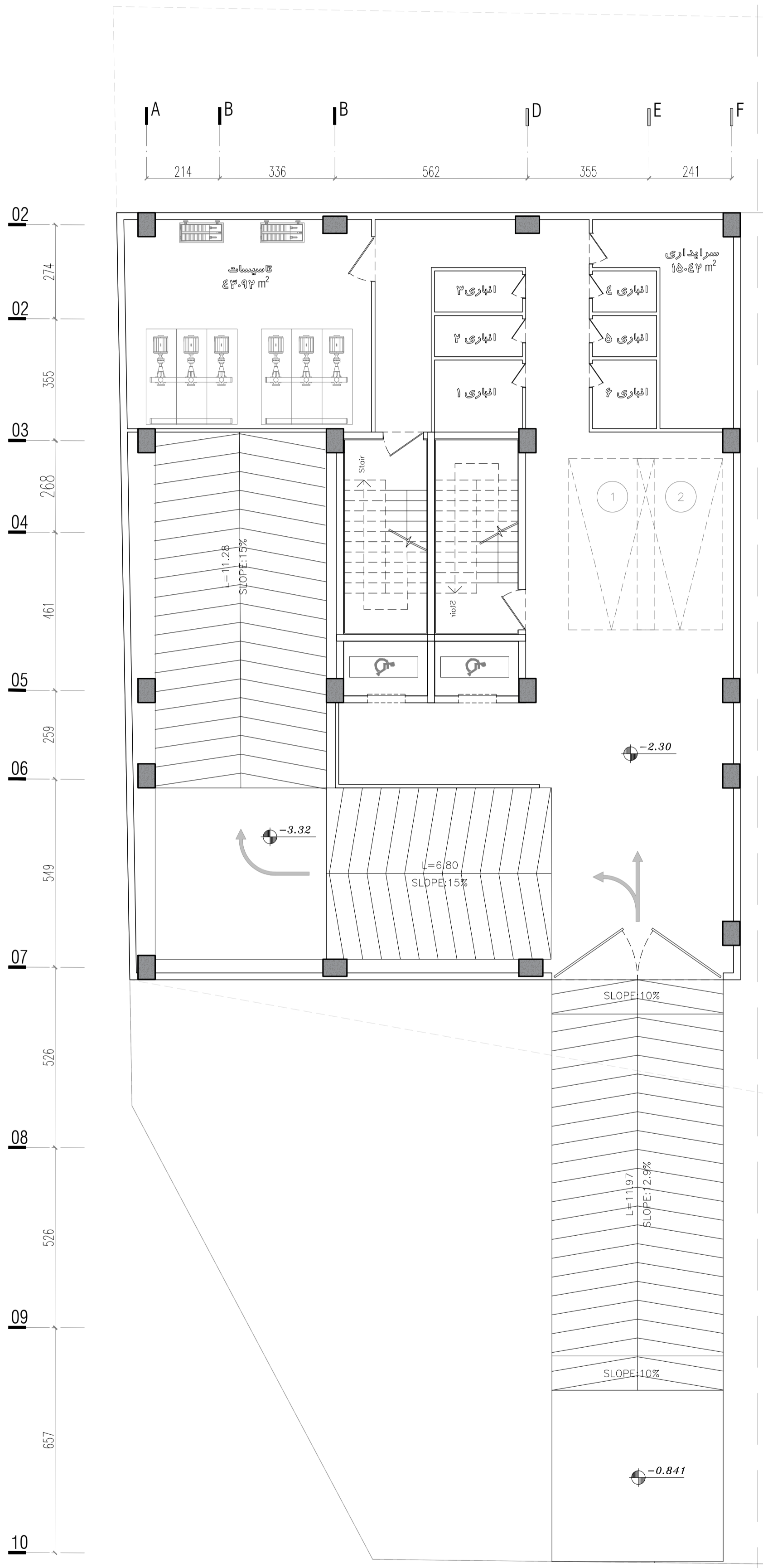
پلان طبقه پارکینگ یکم
