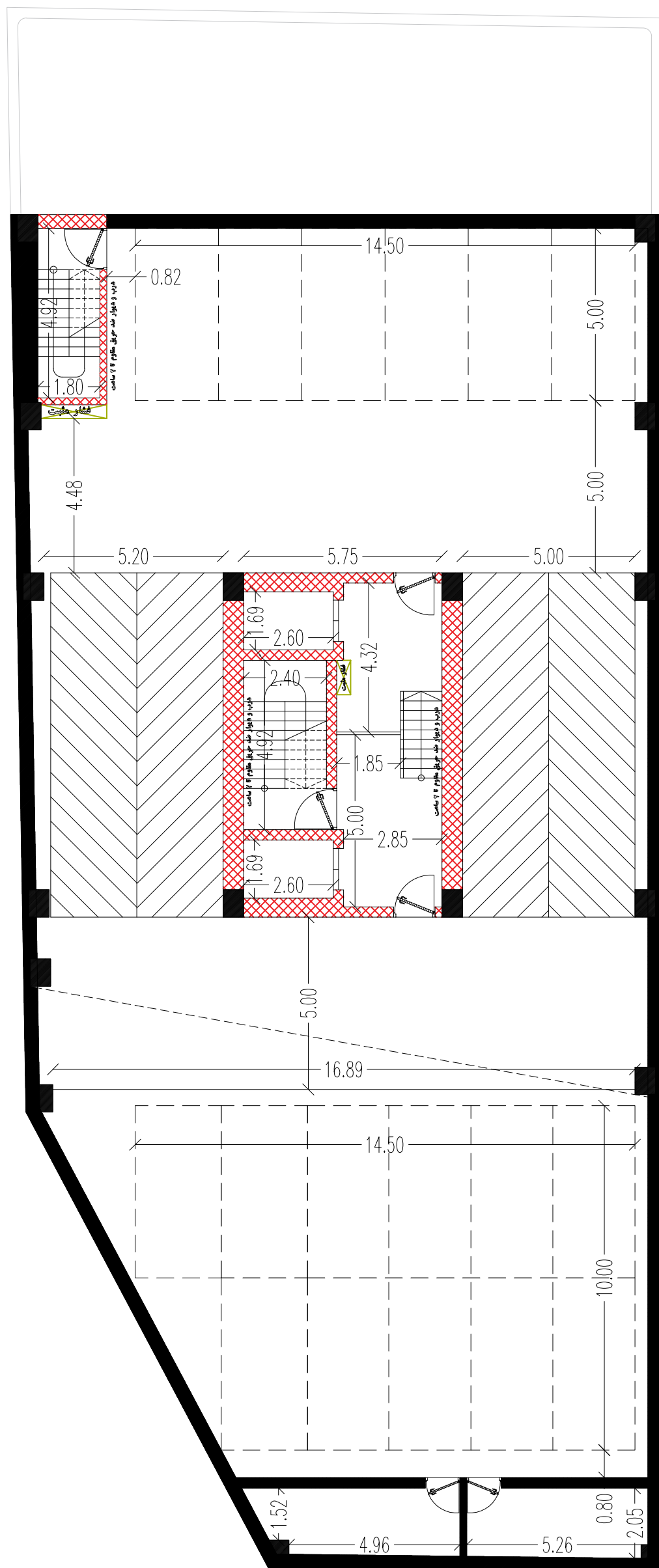
پلان اندازه گذاری زیر زمین چهارم
