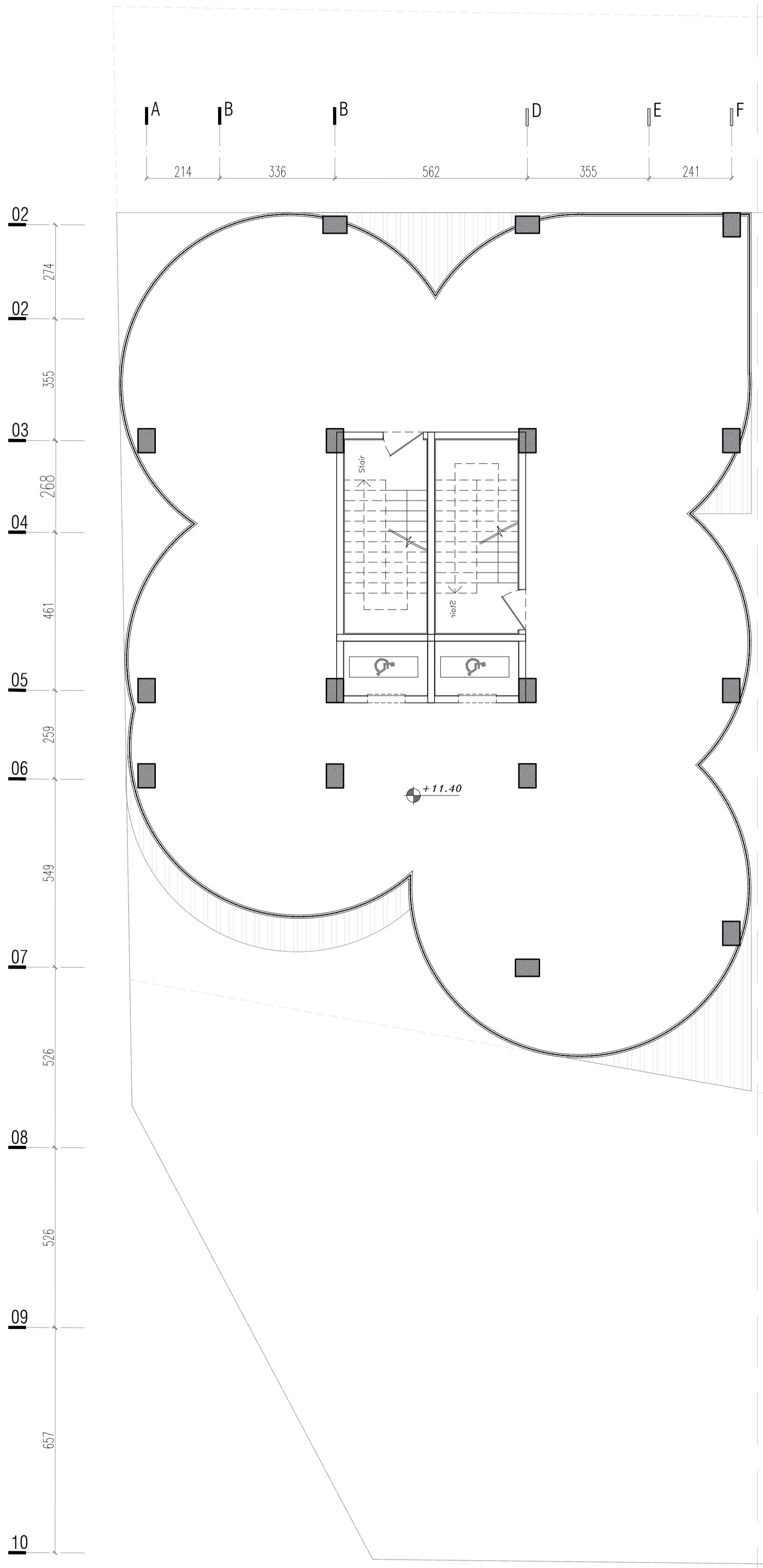
پلان طبقه دوم
