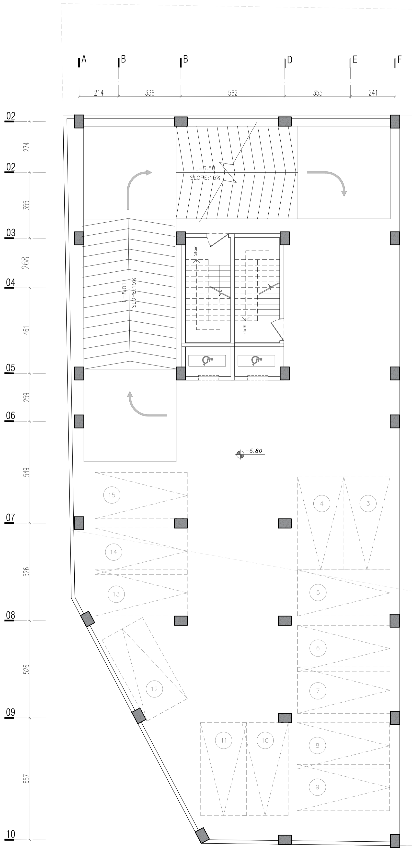
پلان طبقه پارکینگ دوم
