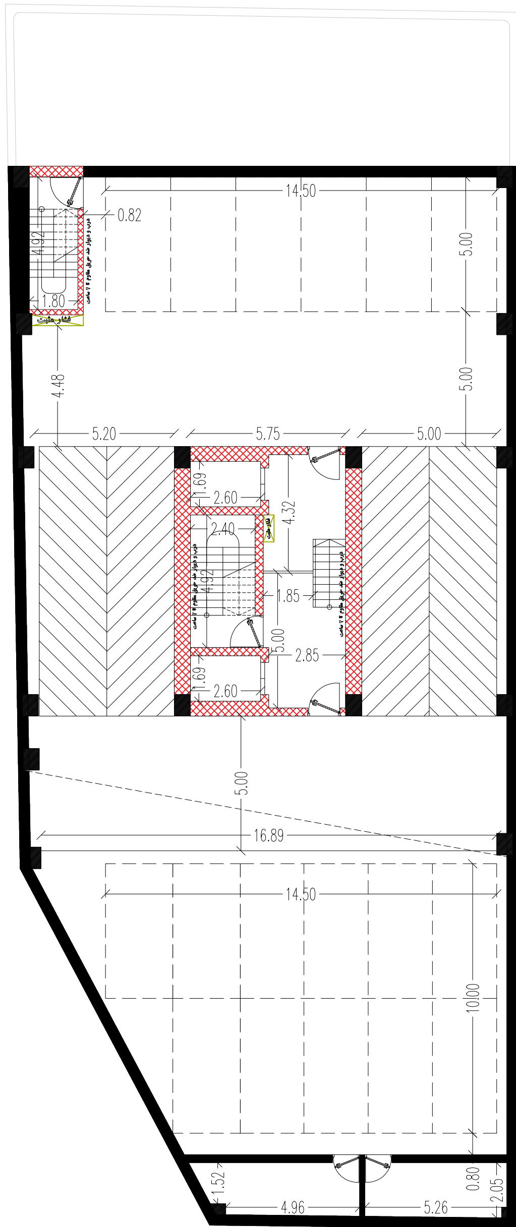
پلان اندازه گذاری زیرزمین سوم
