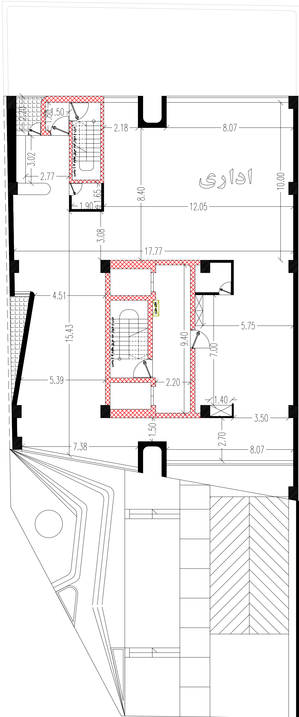
پلان اندازه گذاری طبقه پنجم
