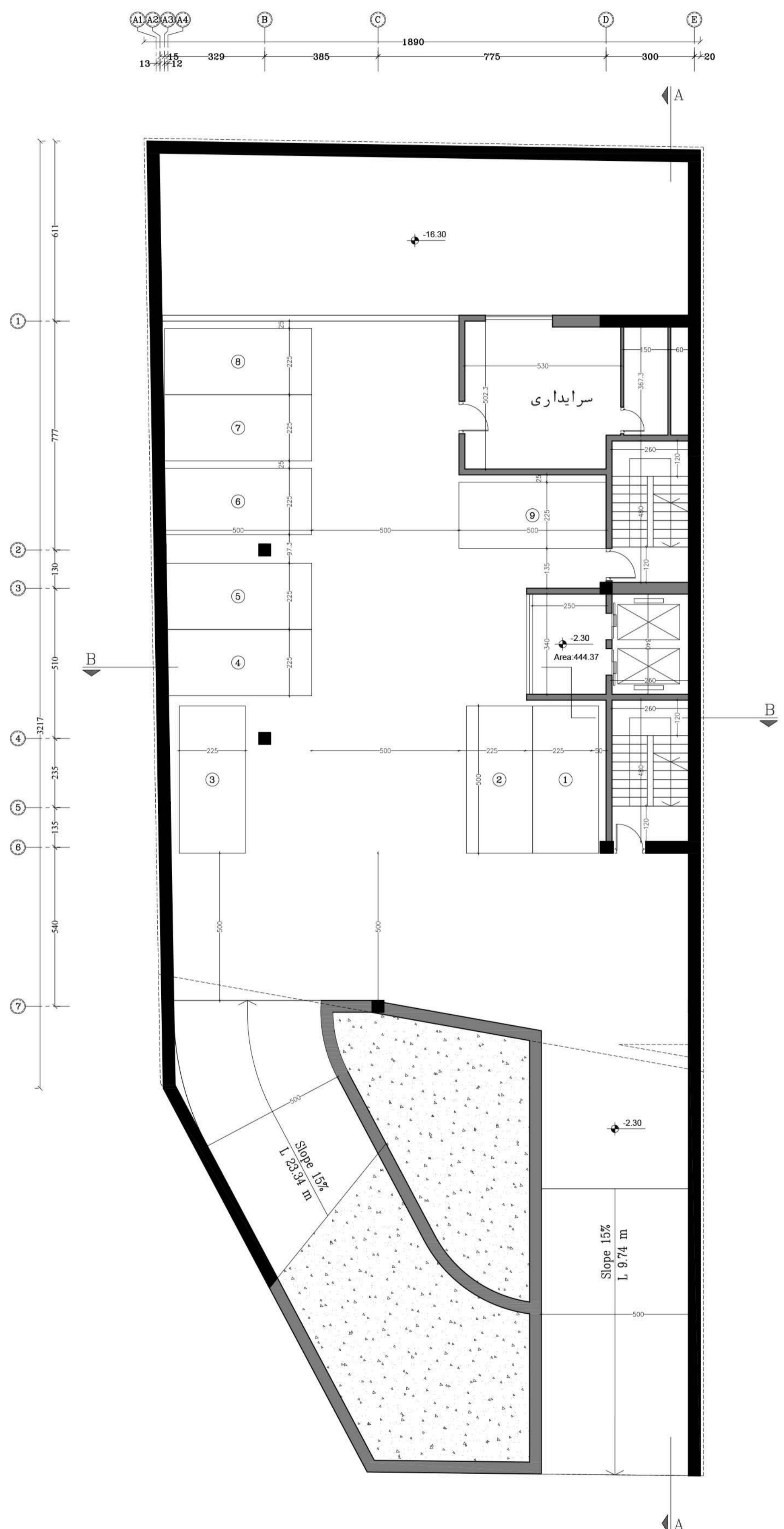
پلان اندازه گذاری گذاری طبقه ۱-
