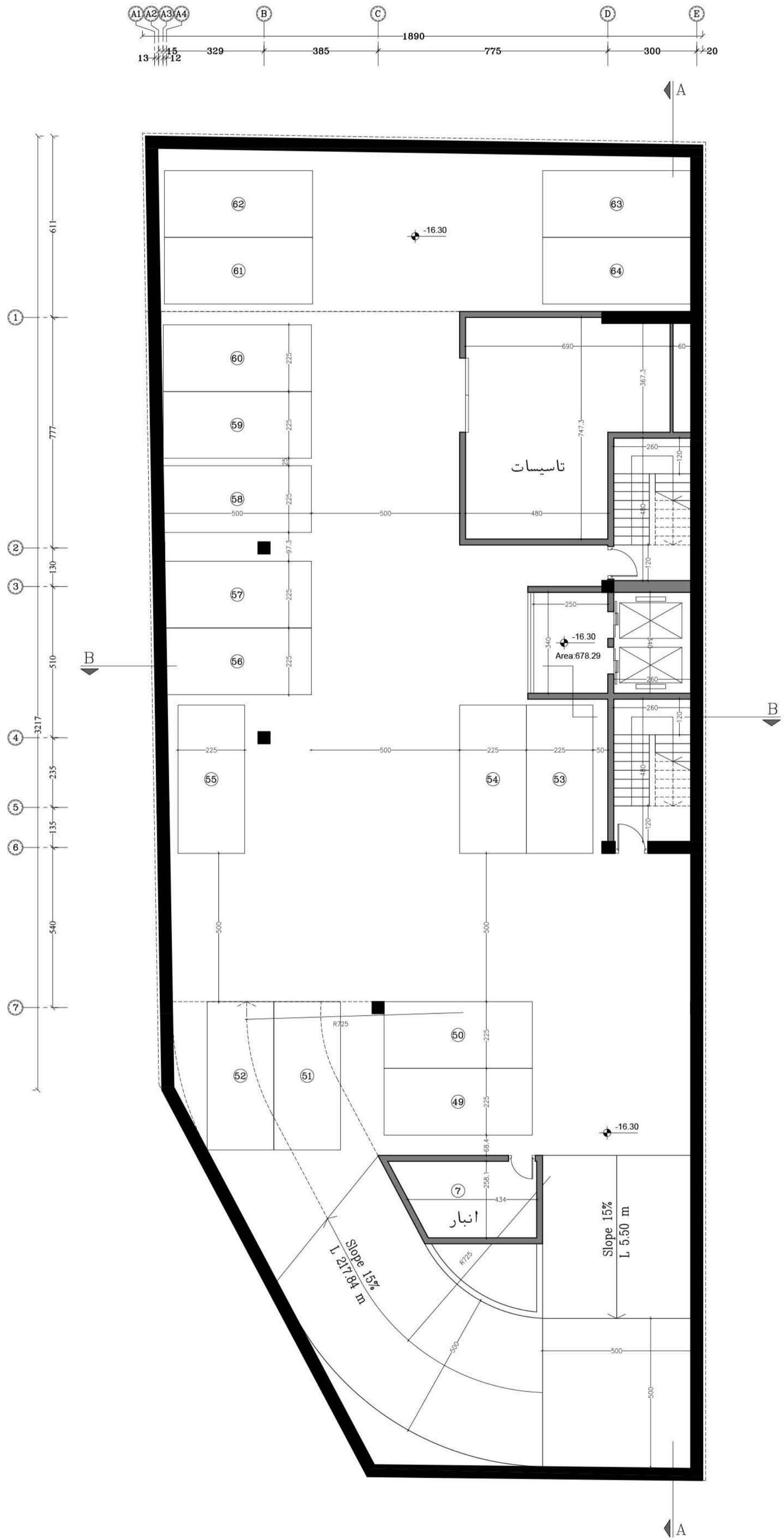
پلان اندازه گذاری طبقه ۵-
