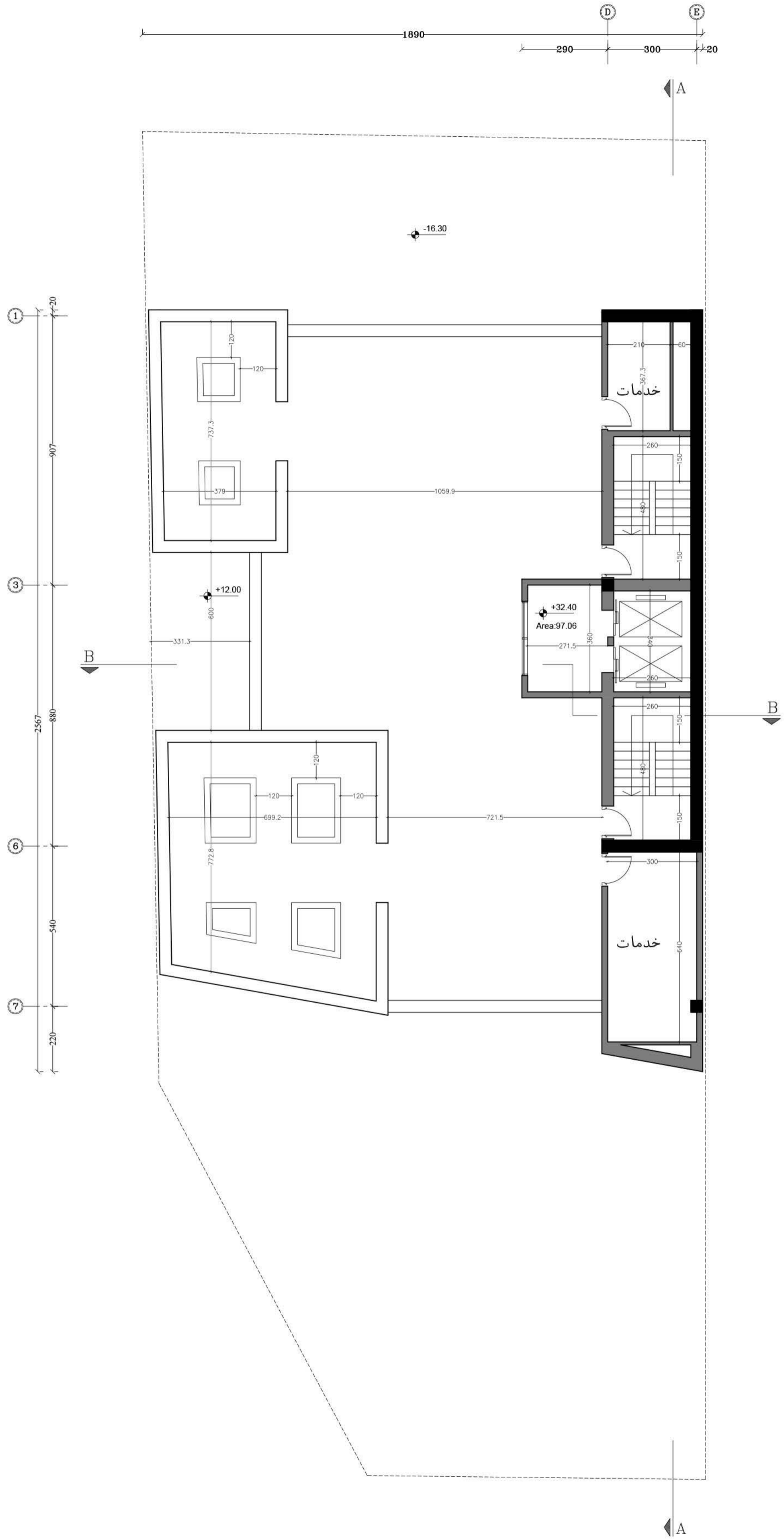
پلان اندازه گذاری گذاری طبقه +۷ (بام)
