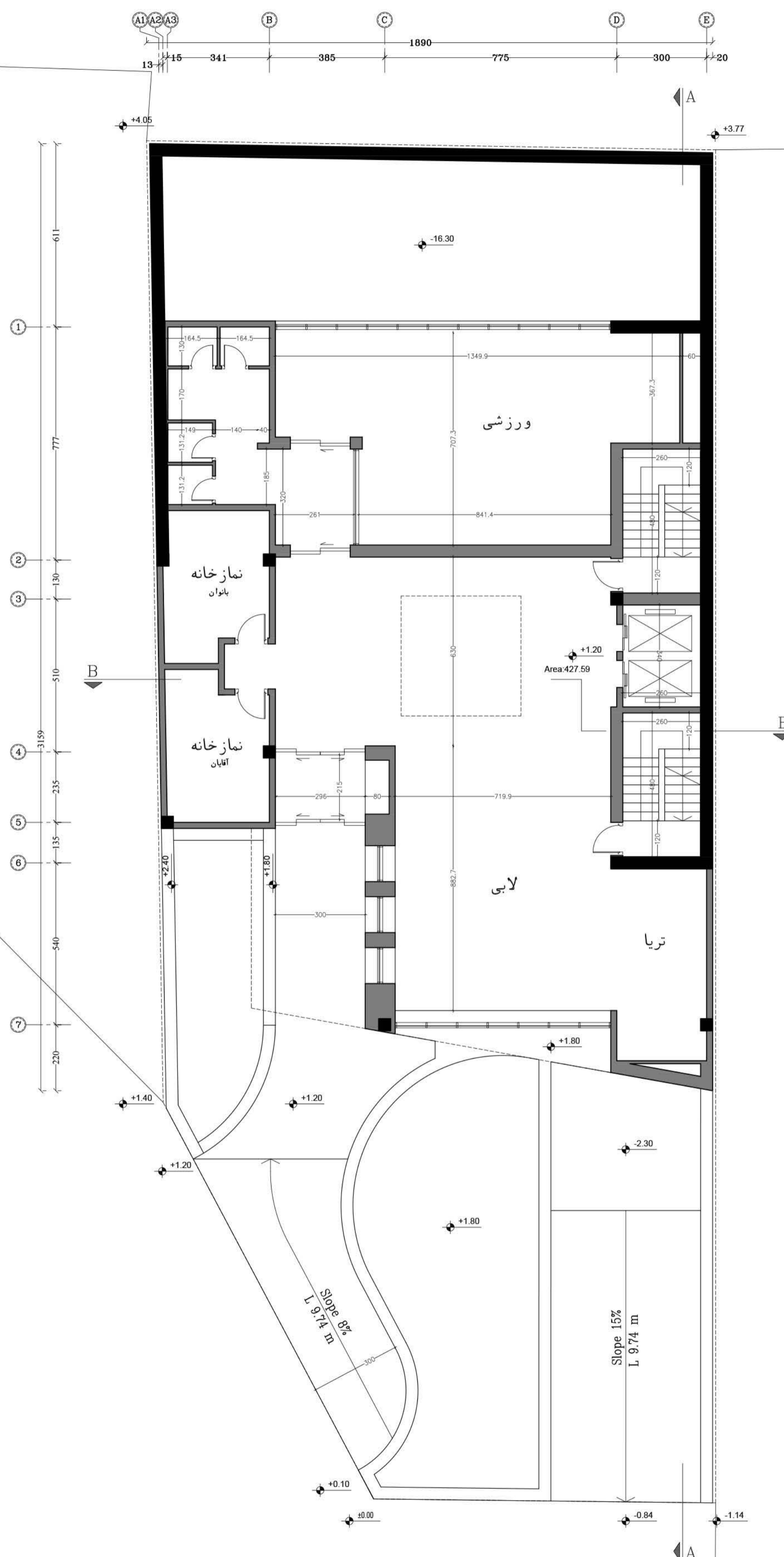
پلان اندازه گذاری طبقه همکف
