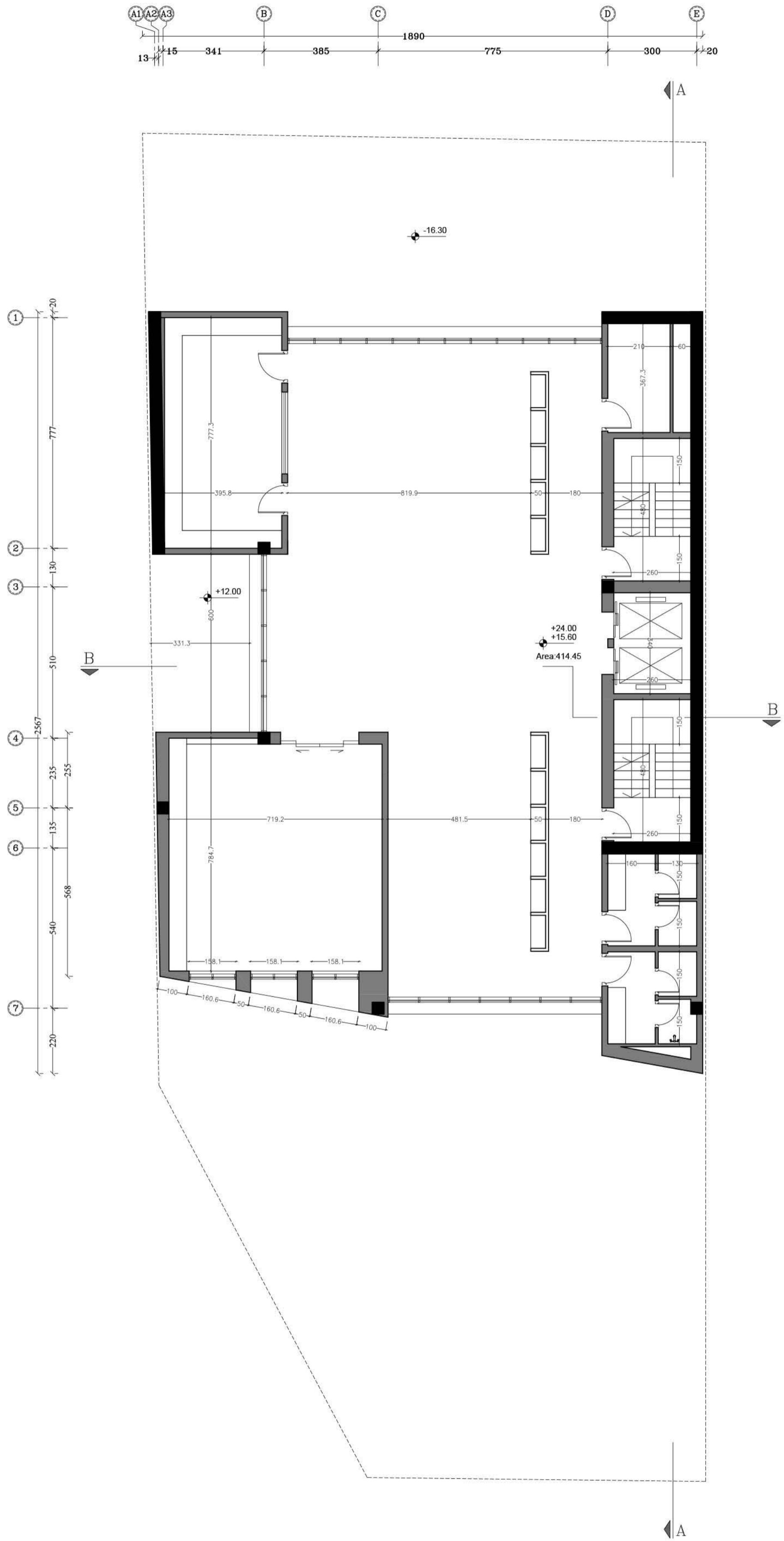
پلان اندازه گذاری گذاری طبقات +۳ ، +۵
