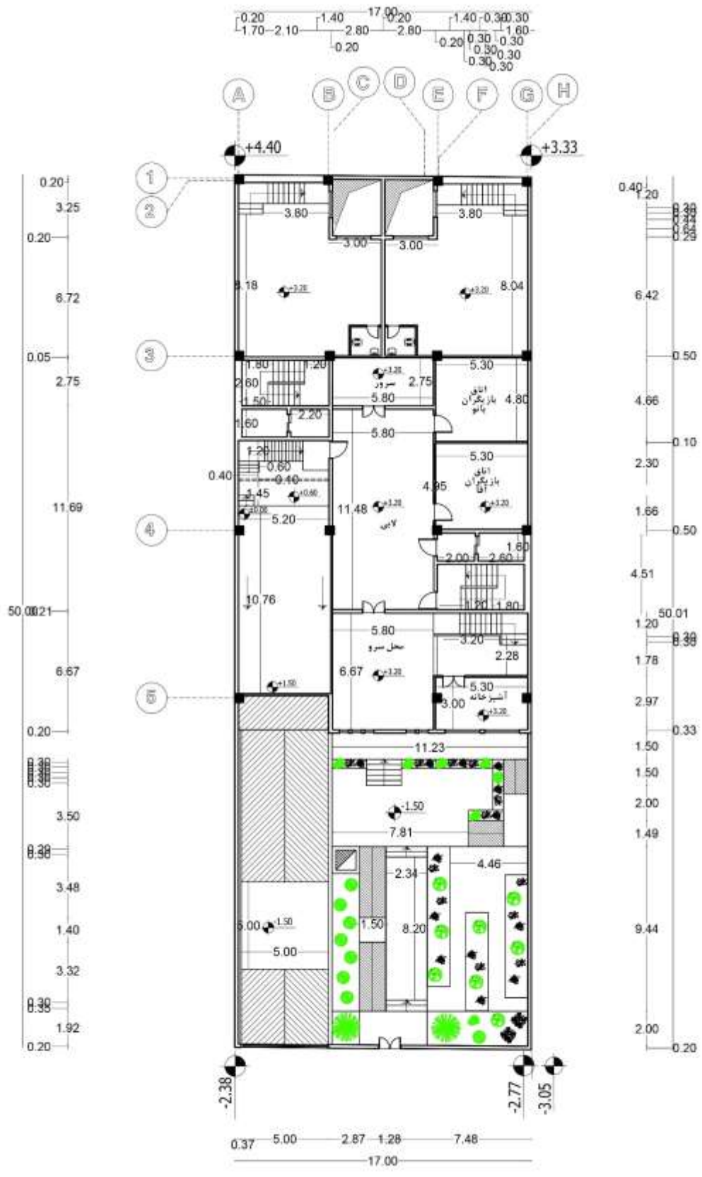
پلان اندازه گذاری نیم طبقه همکف
