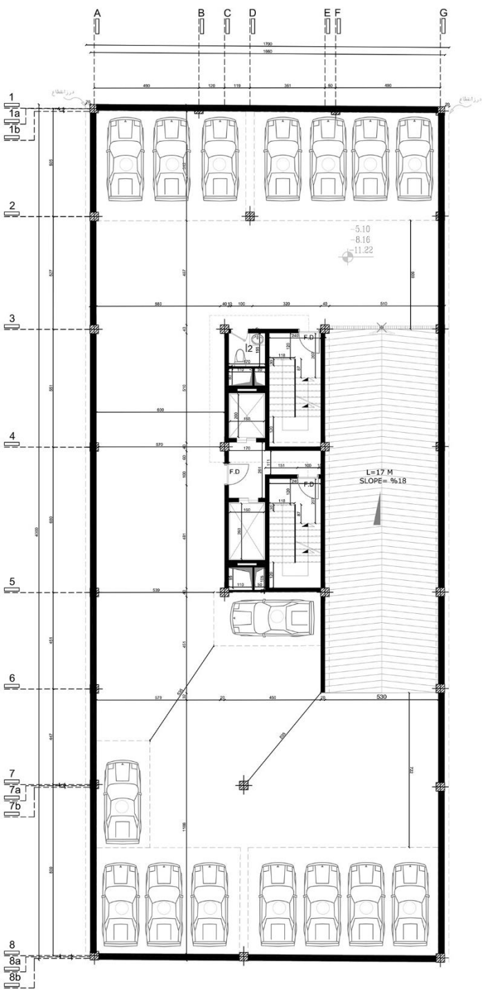
پلان اندازه گذاری طبقات زیرزمین 4، -3، -2
