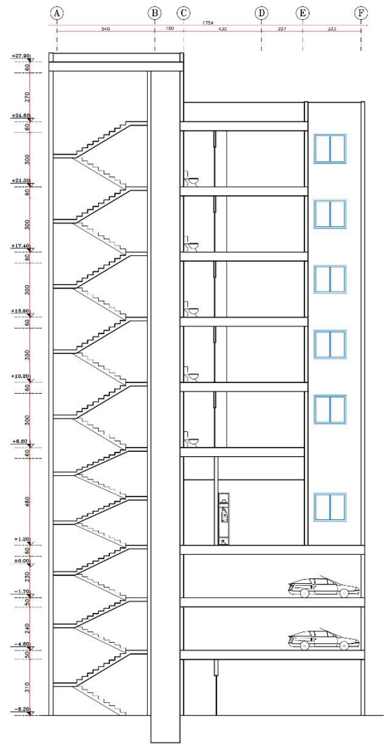
SECTION A-A SC. 1:100
