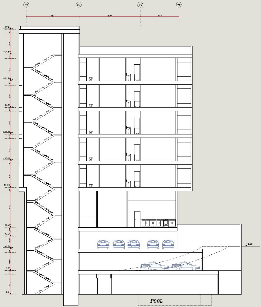
SECTION A-A SC. 1:100
