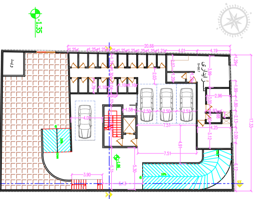
پلان اندازه گذاری زیر زمین اول
