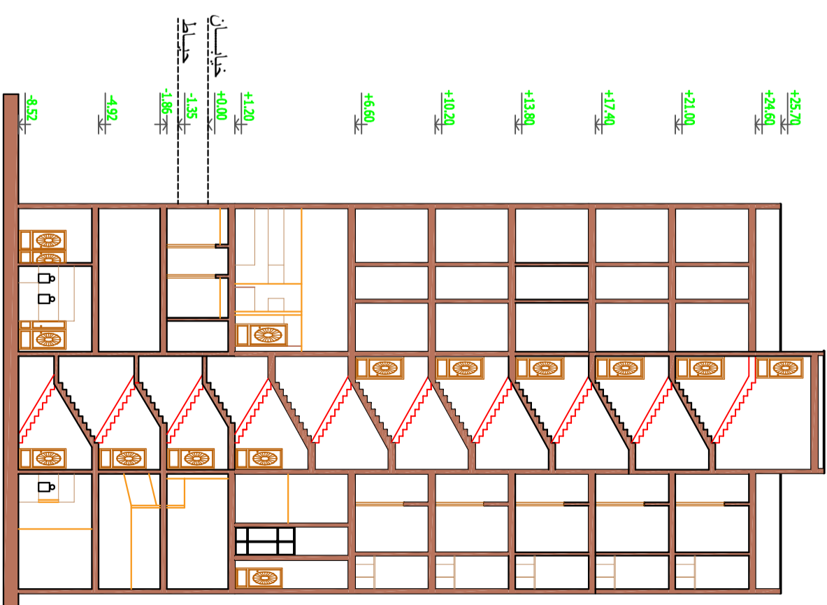
بخش B-B Sc:1:100
