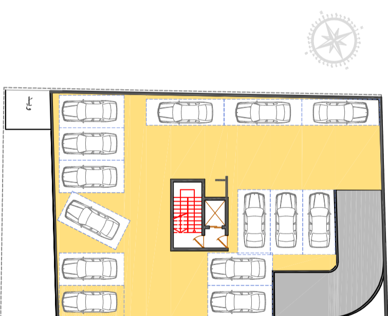
پلان ملبمان زیر زمین دوم
