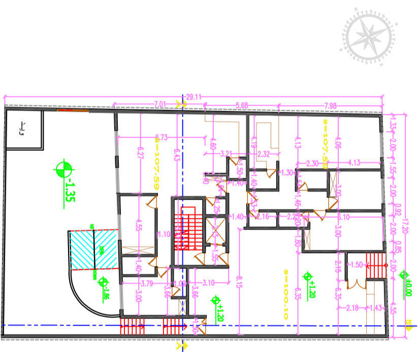
پلان اندازه گذاری همکف
