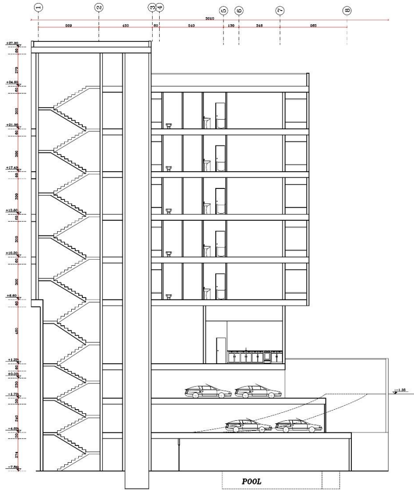
SECTION A-A SC. 1/100
