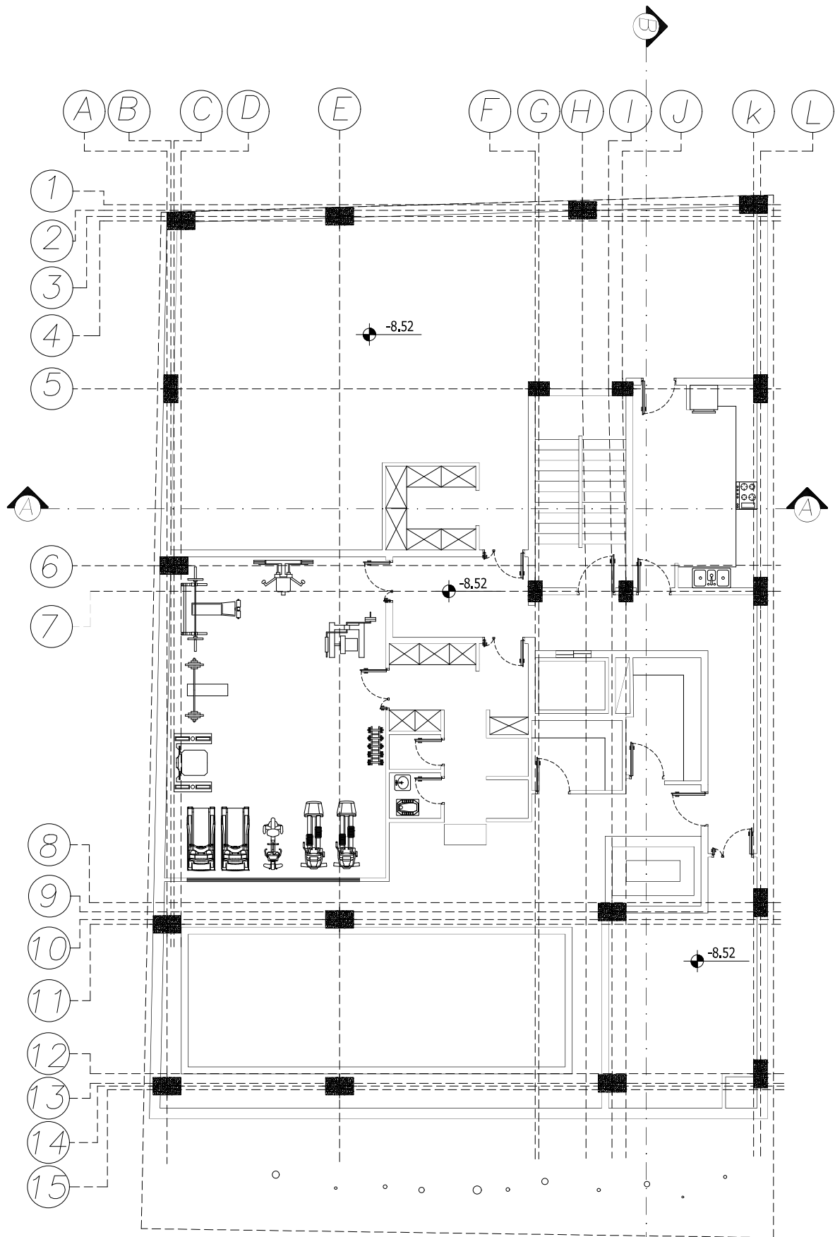
پلان طبقه زیر زمین سوم
