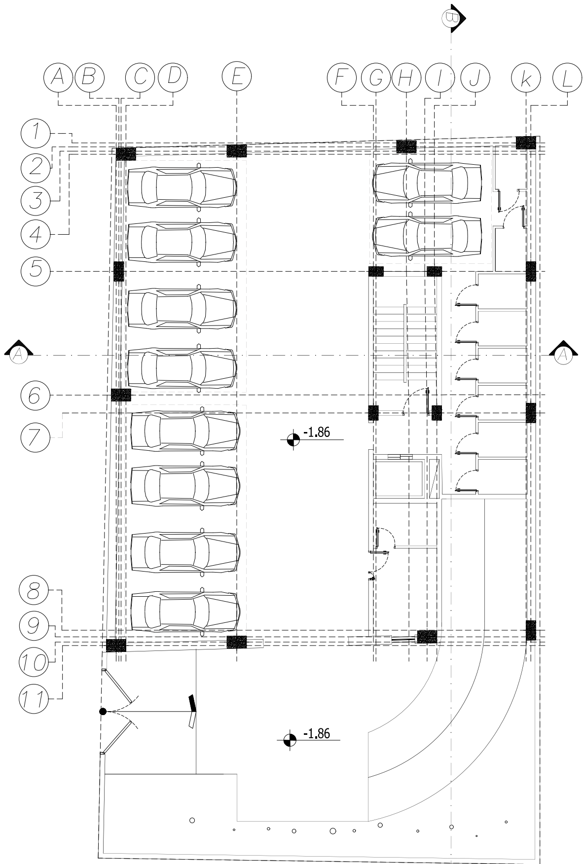
پلان طبقه زیر زمین اول
