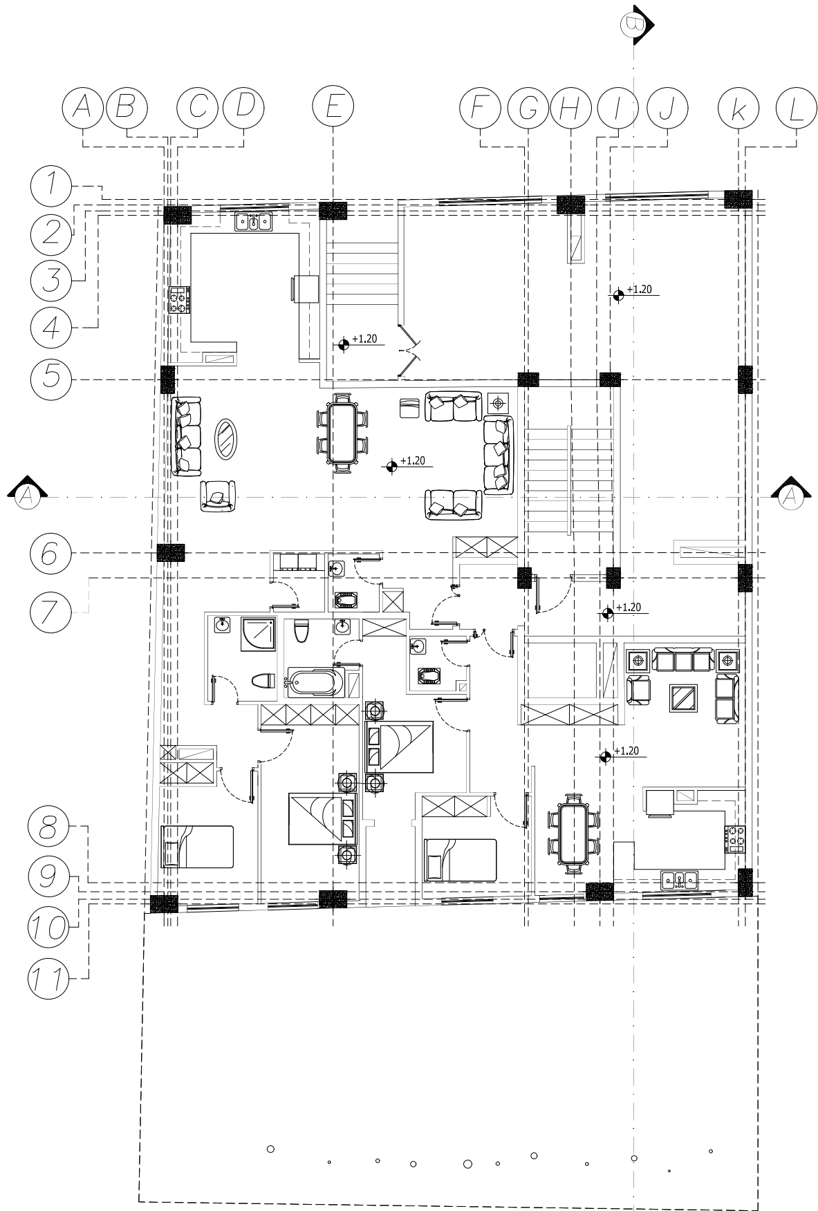
پلان طبقه همکف
