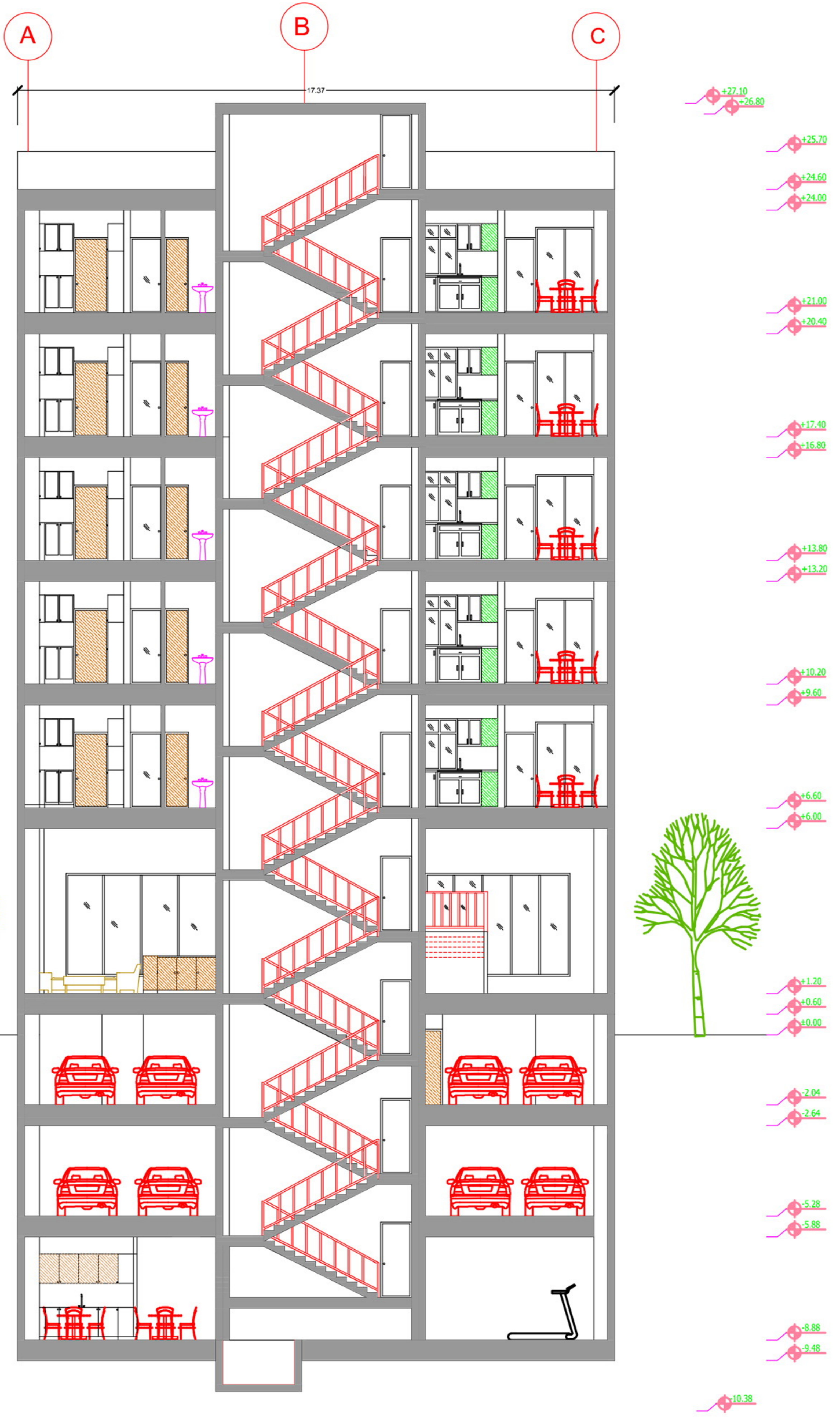
▲ Section-B.B
