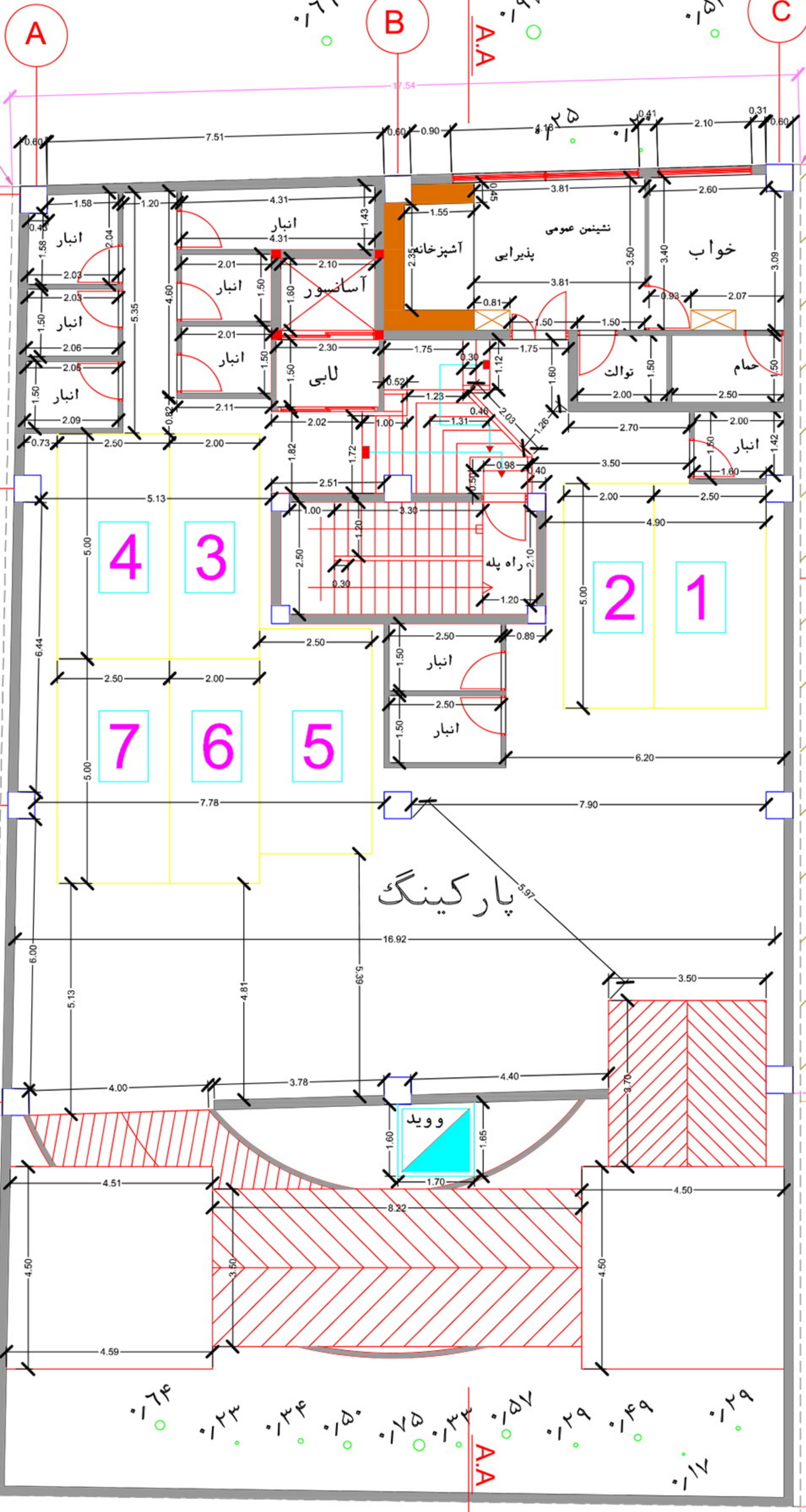
پلان اندازه گذاری طبقه ۱ -
