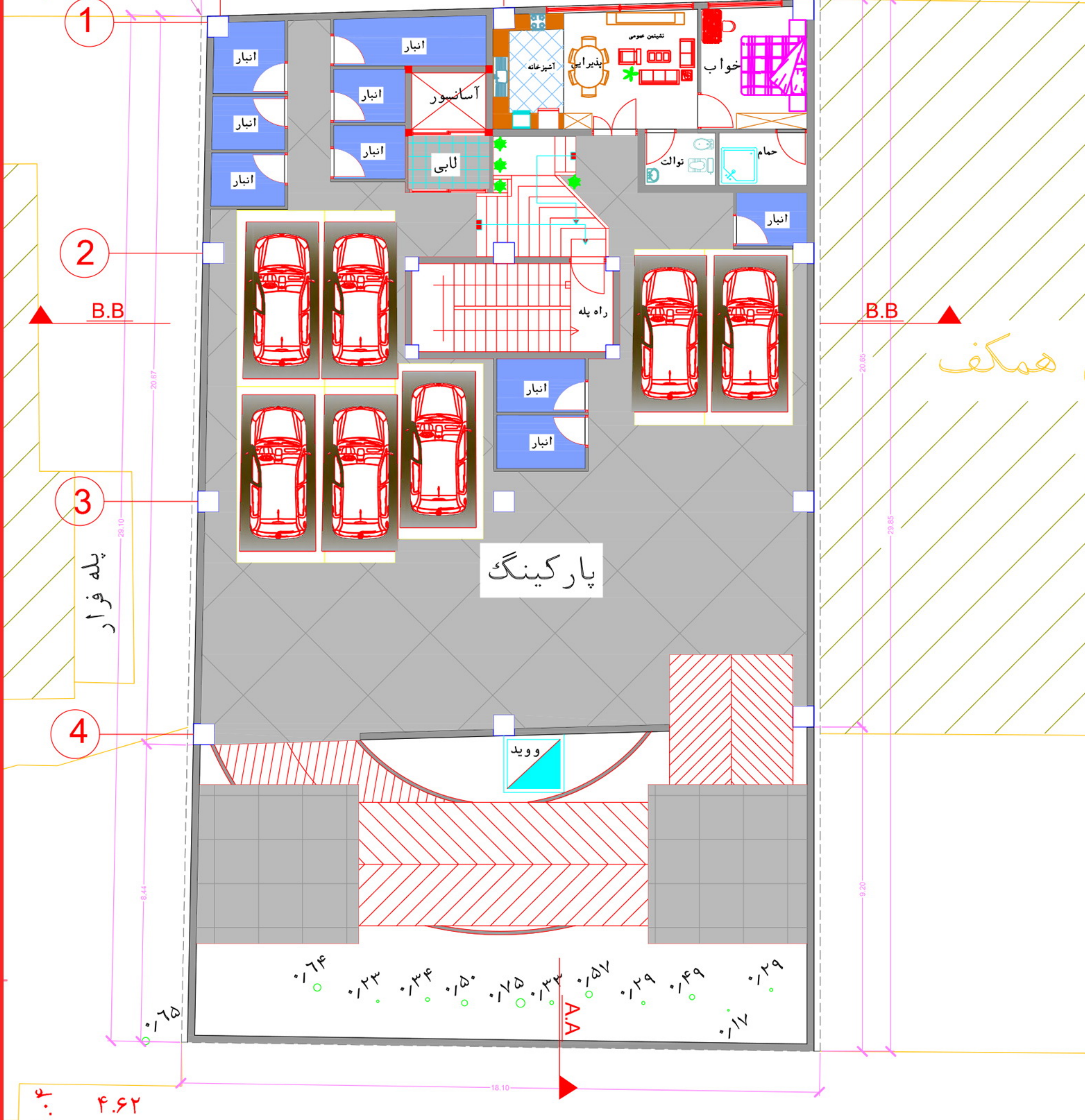
پلان مبلمان طبقه ۱ -
