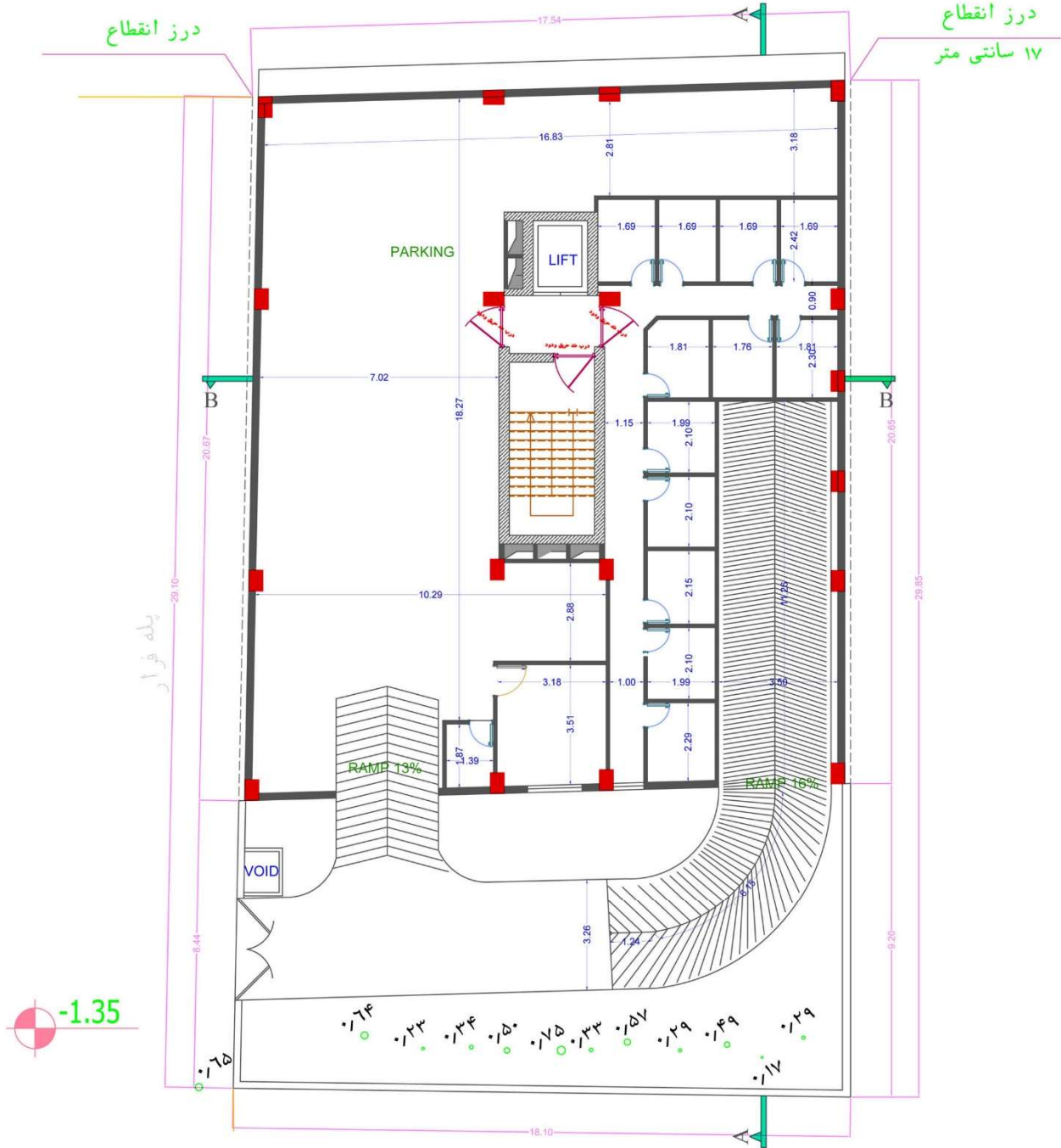
پلان اندازه گذاری زیر زمین ۱
