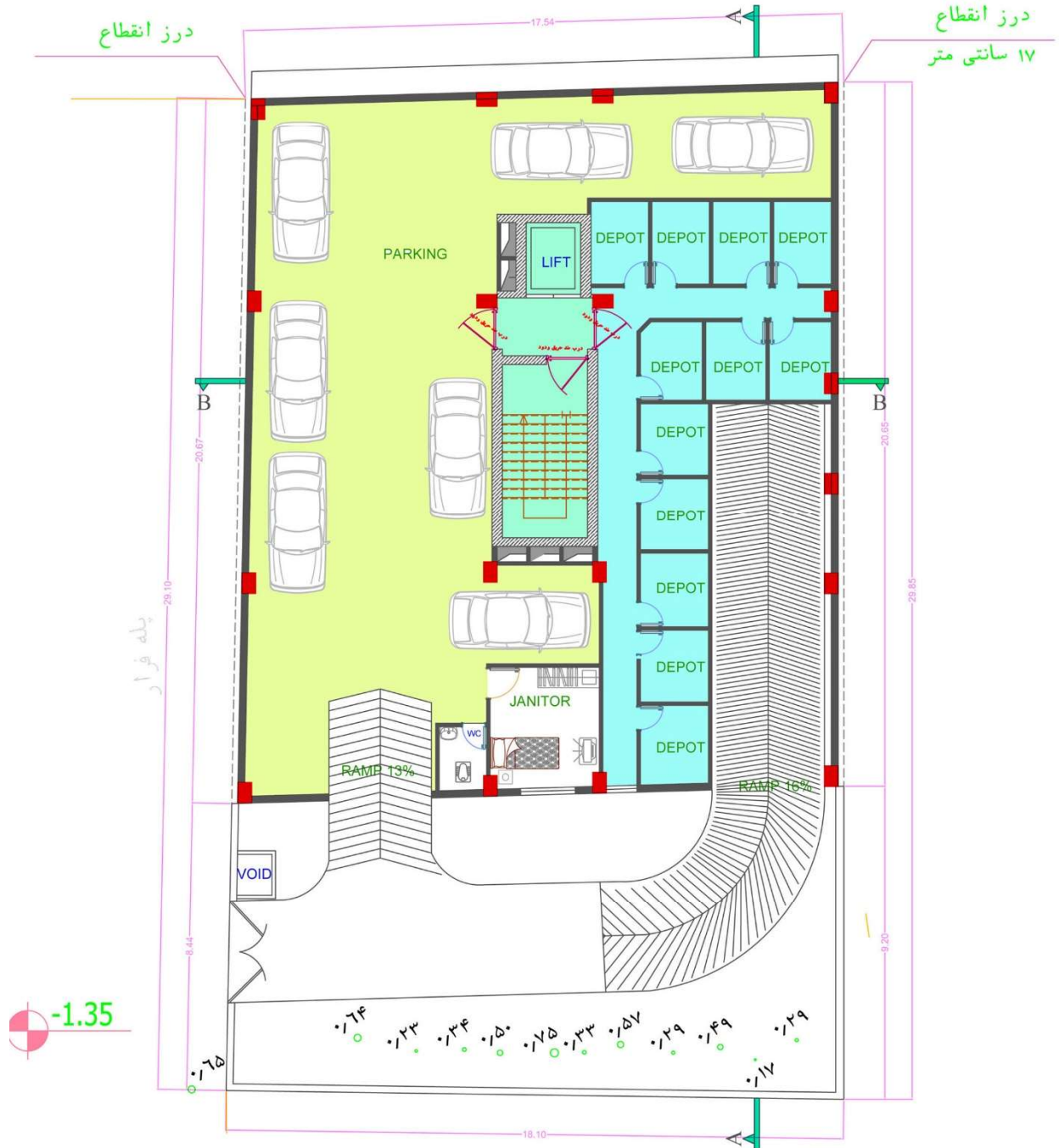
پلان میلمان زیرزمین ۱
