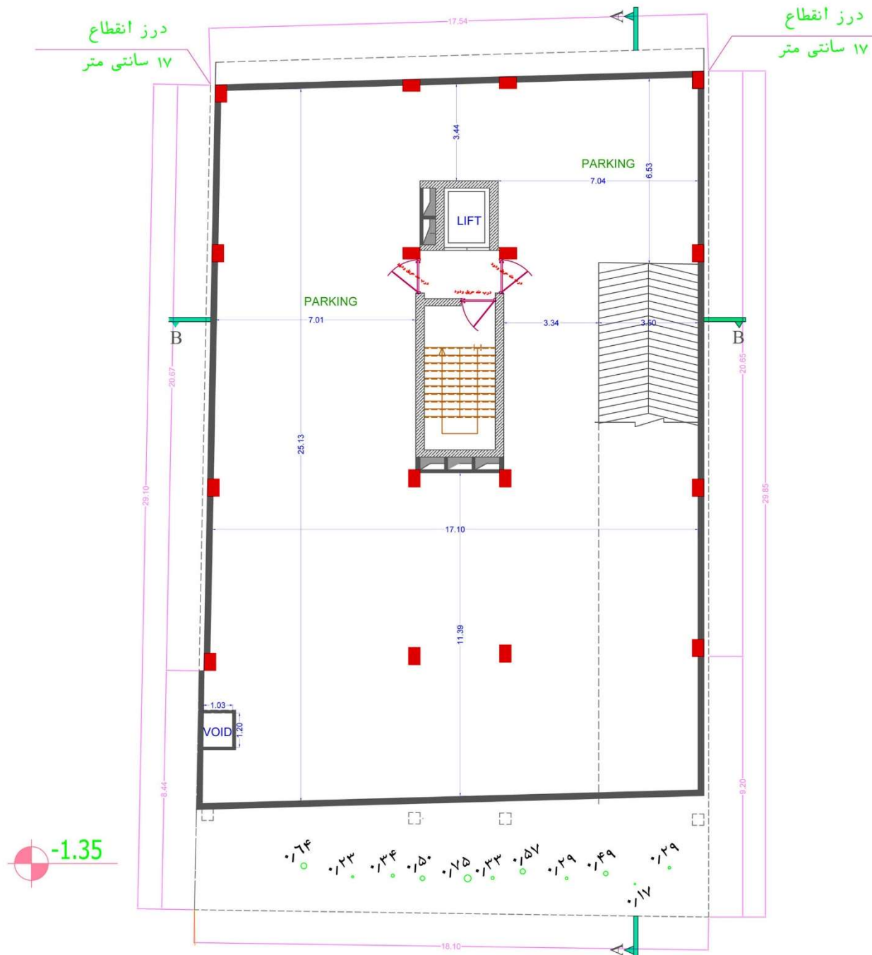
پلان اندازه گذاری زیرزمین ۲
