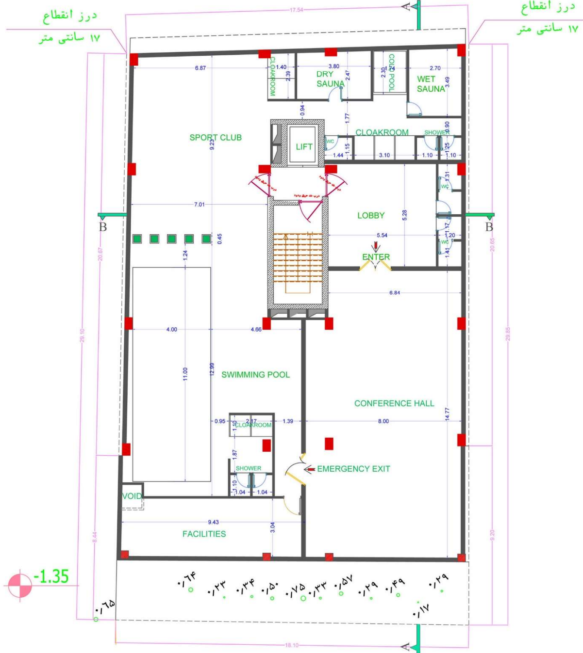
پلان اندازه گذاری زیرزمین ۳
