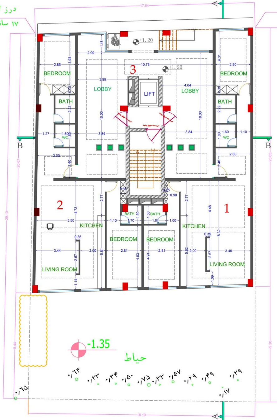
پلان اندازه گذاری طبقه همکف
