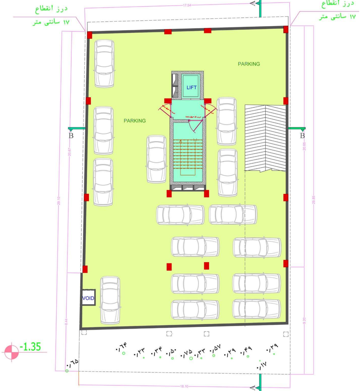
پلان مبلمان زیرزمین ۲
