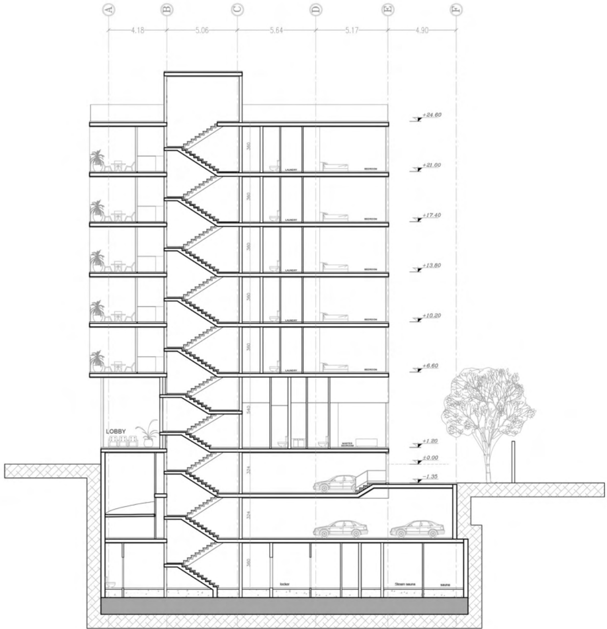
مقطع B-B
