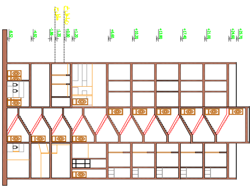
مقطع B-B Scale: 1:100
