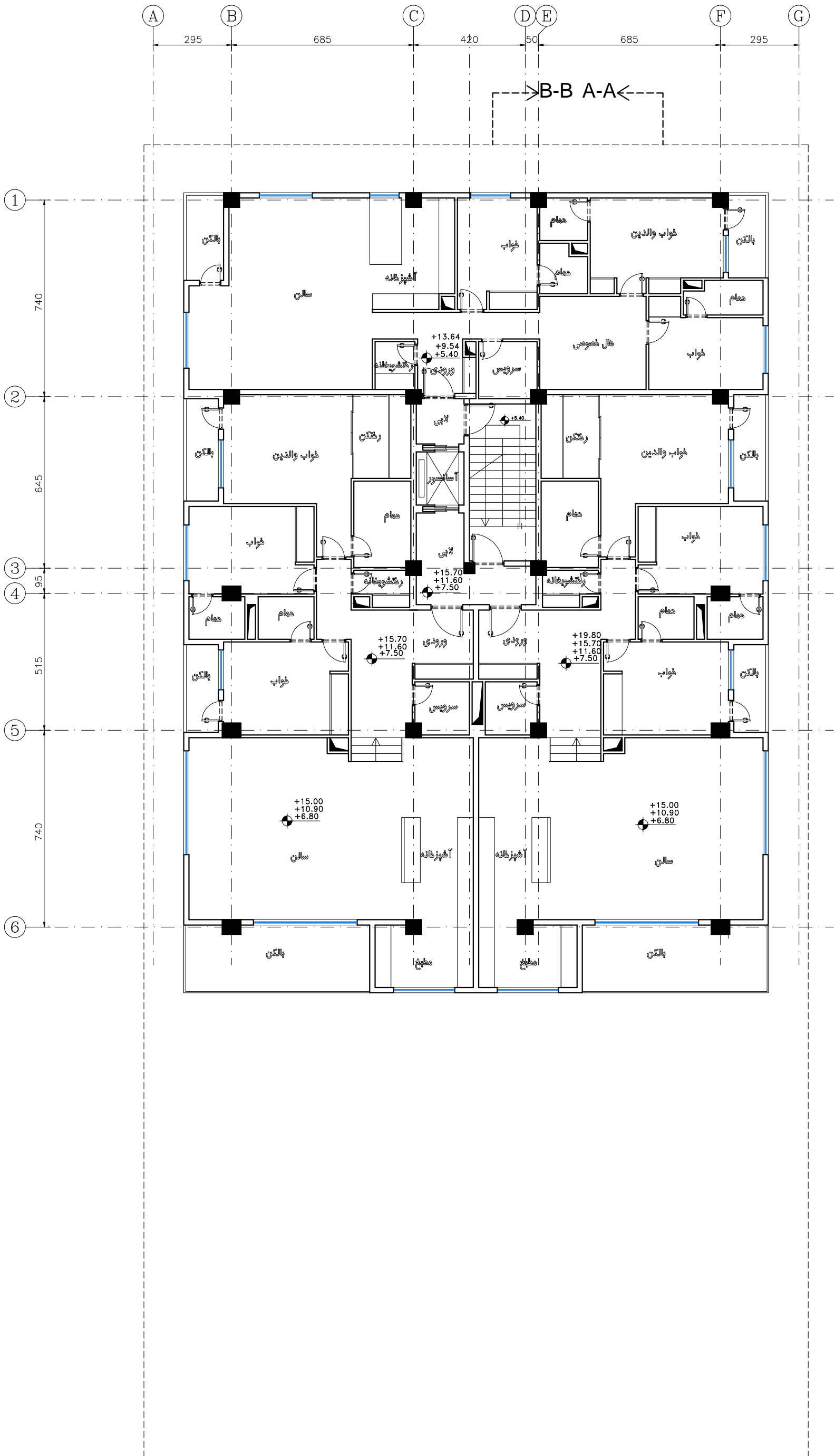
پلان طبقات اول، دوم و سوم
